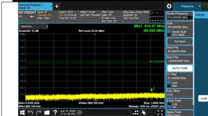
2-2-20MHz-20MHz-QPSK-QPSK-18801-18999-1RB#0-0RB#0-30 ~1000MHz-PASS
