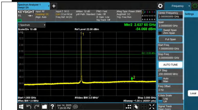
2-2-10MHz-20MHz-QPSK-QPSK-18806-18950-1RB#0-0RB#0-10 00~3000MHz-PASS
