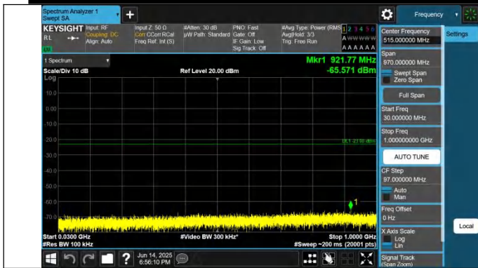
2-2-10MHz-15MHz-QPSK-QPSK-18829-18949-1RB#0-0RB#0-30 ~1000MHz-PASS
