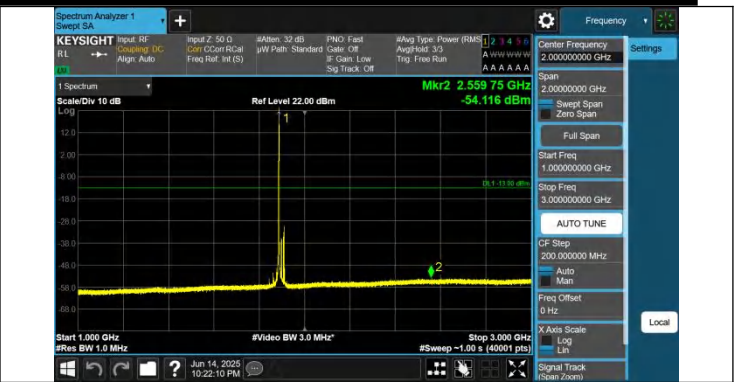
2-2-20MHz-5MHz-QPSK-QPSK-19050-19167-1RB#0-ORB#0-1000~3000MHz-PASS
