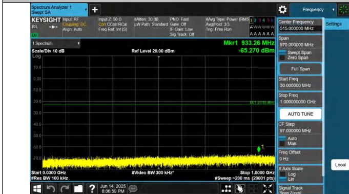
2-2-20MHz-10MHz-QPSK-QPSK-18851-18995-1RB#0-ORB#0-30 ~1000MHz-PASS
