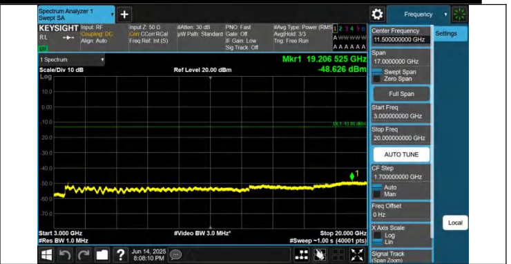
2-2-20MHz-10MHz-QPSK-QPSK-19001-19145-1RB#0-0RB#0-30 00~20000MHz-PASS
