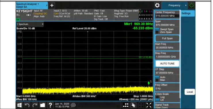
2-2-20MHz-20MHz-QPSK-QPSK-18700-18898-1RB#0-0RB#0-30 ~1000MHz-PASS
