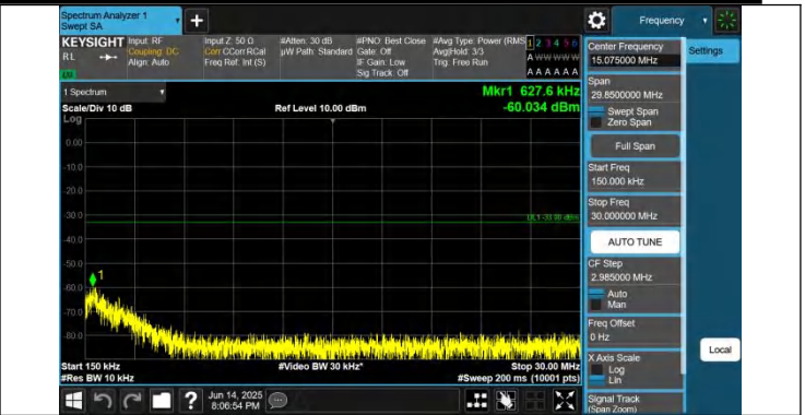
2-2-20MHz-10MHz-QPSK-QPSK-18851-18995-1RB#0-ORB#0-0. 15~30MHz-PASS
