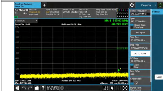
2-2-20MHz-15MHz-QPSK-QPSK-18700-18871-1RB#0-0RB#0-30 ~1000MHz-PASS
