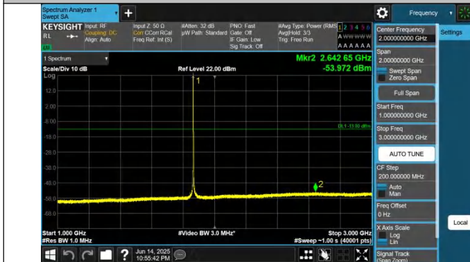
2-2-20MHz-15MHz-QPSK-QPSK-18826-18997-1RB#0-0RB#0-10 00~3000MHz-PASS
