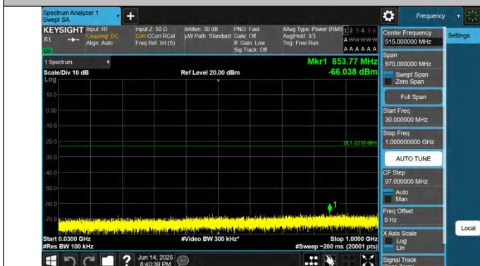
2-2-15MHz-10MHz-QPSK-QPSK-18851-18971-1RB#0-ORB#0-30 ~1000MHz-PASS
