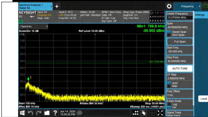
2-2-20MHz-15MHz-QPSK-QPSK-18826-18997-1RB#0-0RB#0-0. 15~30MHz-PASS
