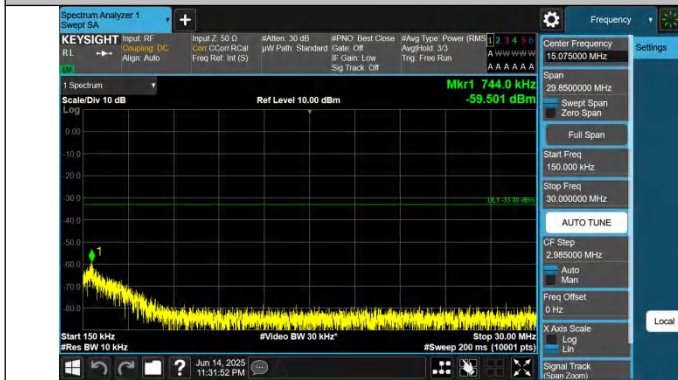
2-2-20MHz-20MHz-QPSK-QPSK-18902-19100-1RB#0-0RB#0-0. 15~30MHz-PASS
