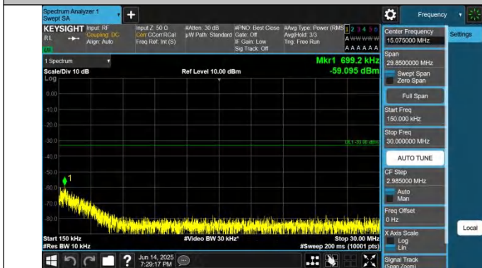
2-2-10MHz-20MHz-QPSK-QPSK-18806-18950-1RB#0-ORB#0-0. 15~30MHz-PASS
