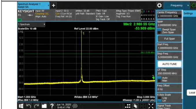
2-2-15MHz-20MHz-QPSK-QPSK-18929-19100-1RB#0-ORB#0-10 00~3000MHz-PASS
