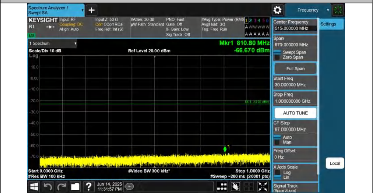
2-2-20MHz-20MHz-QPSK-QPSK-18902-19100-1RB#0-0RB#0-30 ~1000MHz-PASS
