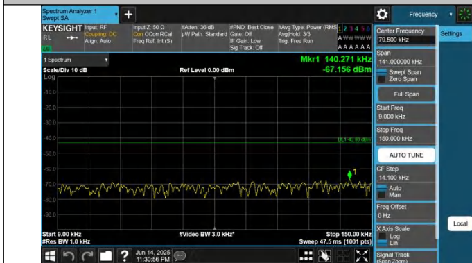
2-2-20MHz-20MHz-QPSK-QPSK-18801-18999-1RB#0-0RB#0-0. 009~0.15MHz-PASS
