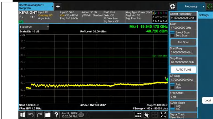
2-2-20MHz-5MHz-QPSK-QPSK-18700-18817-1RB#0-ORB#0-300 0~20000MHz-PASS
