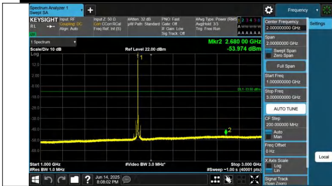
2-2-20MHz-10MHz-QPSK-QPSK-19001-19145-1RB#0-0RB#0-10 00~3000MHz-PASS
