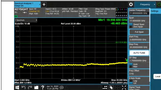
2-2-20MHz-20MHz-QPSK-QPSK-18801-18999-1RB#0-0RB#0-30 00~20000MHz-PASS
