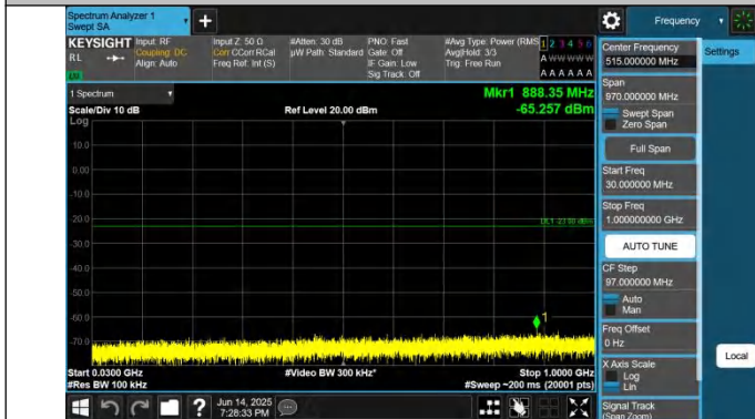
2-2-10MHz-20MHz-QPSK-QPSK-18655-18799-1RB#0-ORB#0-30 ~1000MHz-PASS
