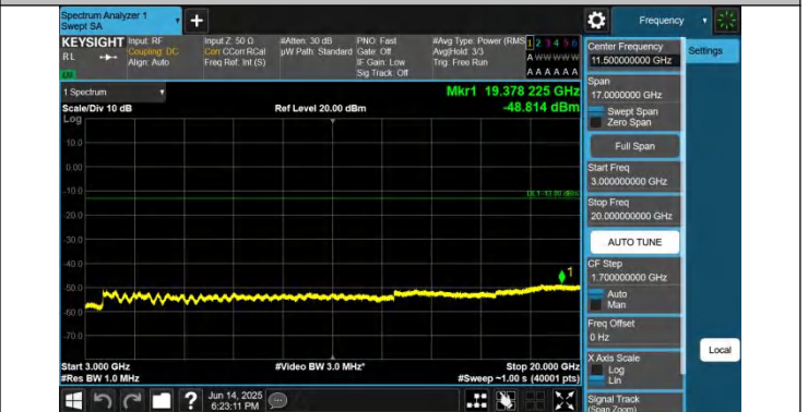
2-2-5MHz-20MHz-QPSK-QPSK-18808-18925-1RB#0-ORB#0-300 0~20000MHz-PASS
