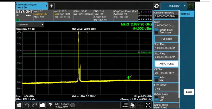
2-2-10MHz-15MHz-QPSK-QPSK-18829-18949-1RB#0-0RB#0-10 00~3000MHz-PASS
