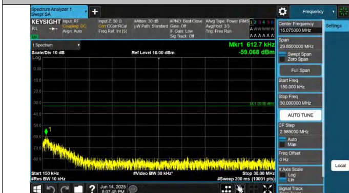
2-2-20MHz-10MHz-QPSK-QPSK-19001-19145-1RB#0-ORB#0-0. 15~30MHz-PASS
