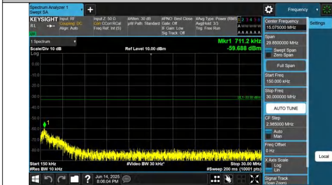
2-2-20MHz-10MHz-QPSK-QPSK-18700-18844-1RB#0-ORB#0-0.15~30MHz-PASS
