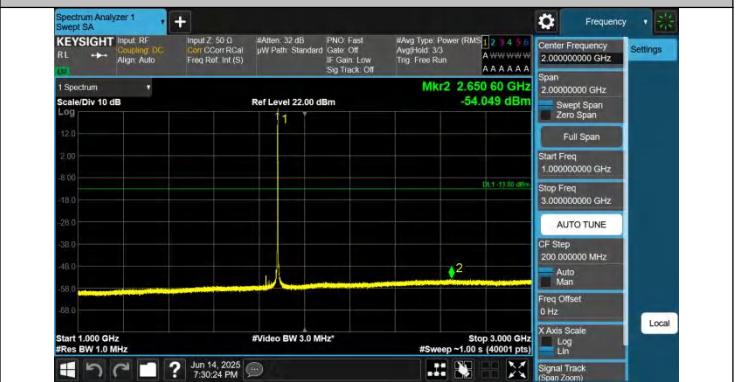
2-2-10MHz-20MHz-QPSK-QPSK-18956-19100-1RB#0-0RB#0-10 00~3000MHz-PASS
