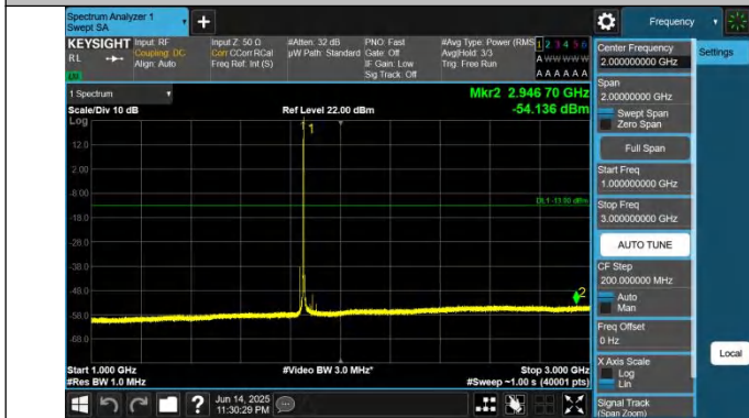
2-2-20MHz-20MHz-QPSK-QPSK-18700-18898-1RB#0-0RB#0-10 00~3000MHz-PASS
