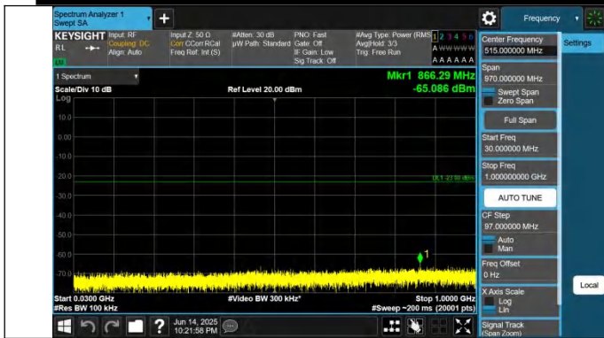
2-2-20MHz-5MHz-QPSK-QPSK-19050-19167-1RB#0-ORB#0-30~1000MHz-PASS
