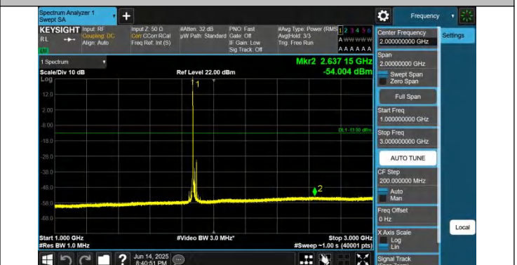
2-2-15MHz-10MHz-QPSK-QPSK-18851-18971-1RB#0-ORB#0-10 00~3000MHz-PASS
