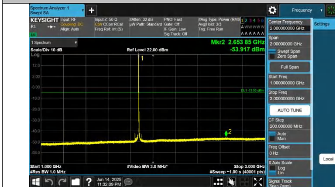
2-2-20MHz-20MHz-QPSK-QPSK-18902-19100-1RB#0-0RB#0-10 00~3000MHz-PASS
