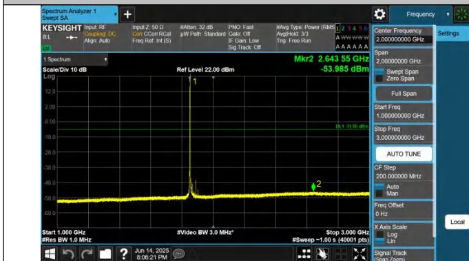
2-2-20MHz-10MHz-QPSK-QPSK-18700-18844-1RB#0-ORB#0-1000~3000MHz-PASS
