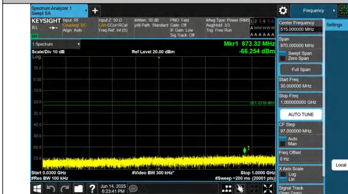
2-2-5MHz-20MHz-QPSK-QPSK-18983-19100-1RB#0-ORB#0-30~ 1000MHz-PASS
