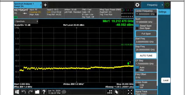
2-2-20MHz-20MHz-QPSK-QPSK-18700-18898-1RB#0-0RB#0-30 00~20000MHz-PASS
