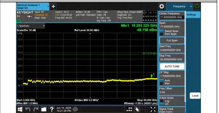
2-2-20MHz-5MHz-QPSK-QPSK-18875-18992-1RB#0-ORB#0-300 0~20000MHz-PASS
