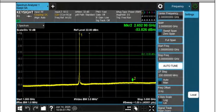
2-2-20MHz-15MHz-QPSK-QPSK-18700-18871-1RB#0-0RB#0-10 00~3000MHz-PASS
