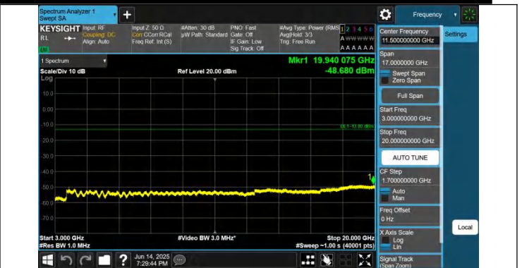
2-2-10MHz-20MHz-QPSK-QPSK-18806-18950-1RB#0-0RB#0-30 00~20000MHz-PASS
