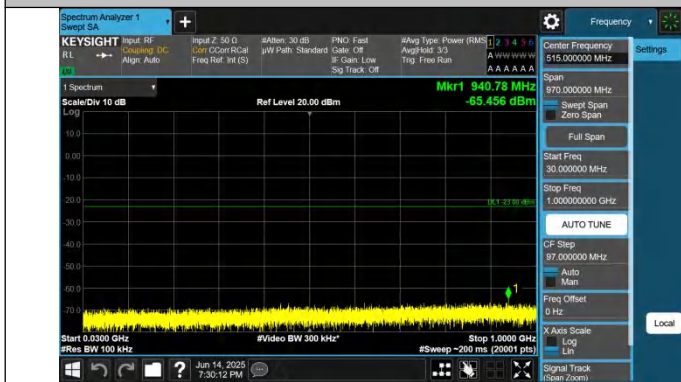
2-2-10MHz-20MHz-QPSK-QPSK-18956-19100-1RB#0-0RB#0-30 ~1000MHz-PASS
