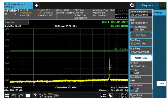
Band26(824-849)-3MHz-QPSK-27025-1RB#0-30~1000-PASS
