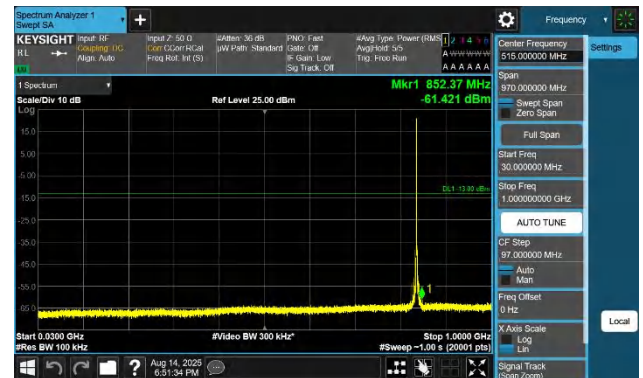
Band26(824-849)-10MHz-QPSK-26990-1RB#0-30~1000-PASS
