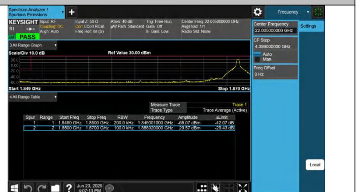
Band25-20MHz-QPSK-26140-1RB#99-PASS
