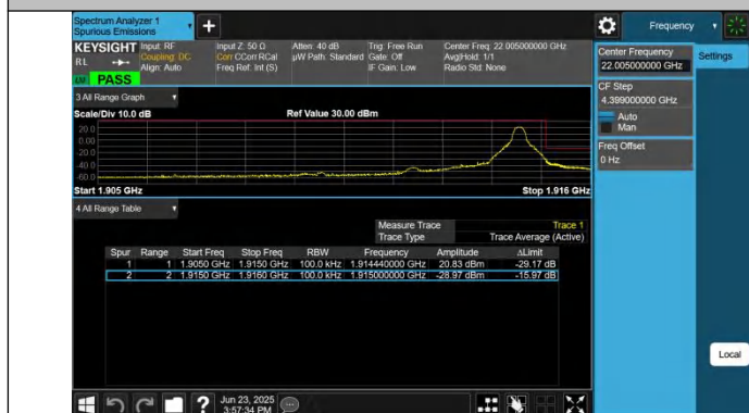
Band25-10MHz-QPSK-26640-1RB#0-PASS
