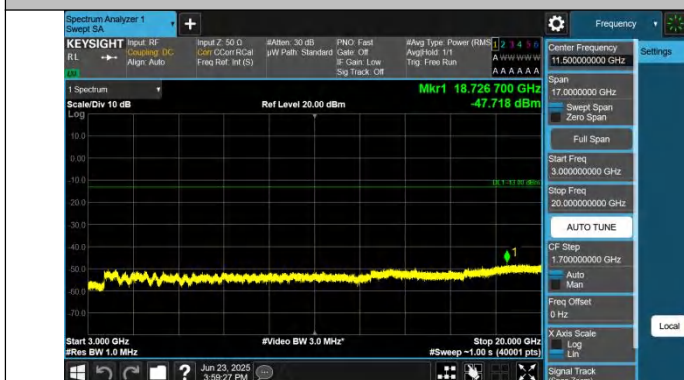
Band25-10MHz-QPSK-26365-1RB#0-3000~20000-PASS
