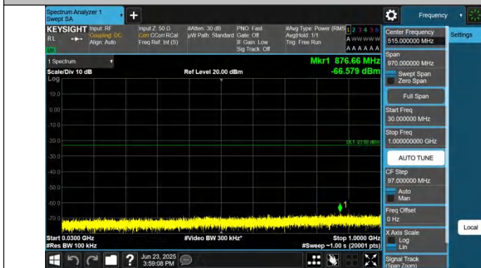
Band25-10MHz-QPSK-26365-1RB#0-30~1000-PASS
