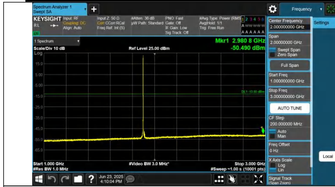
Band25-20MHz-QPSK-26590-1RB#0-1000~3000-PASS
