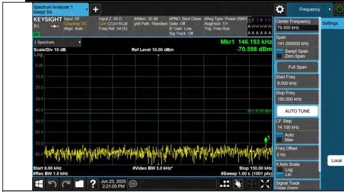
Band4-20MHz-QPSK-20175-1RB#0-0.009~0.15-PASS
