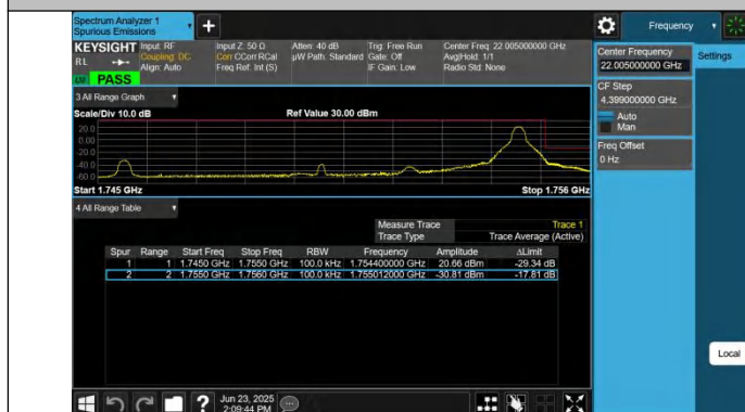
Band4-10MHz-QPSK-20350-1RB#49-PASS
