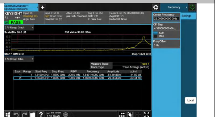
Band2-20MHz-QPSK-18700-1RB#99-PASS
