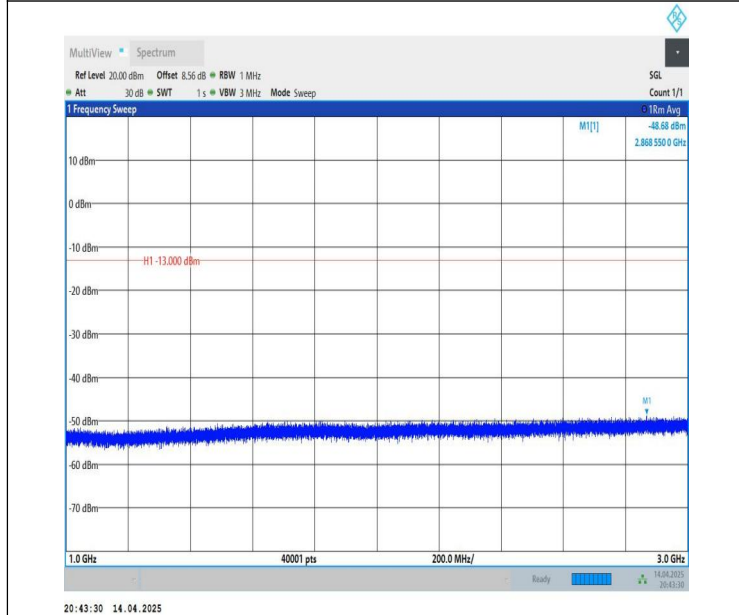
Band26(824-849)-10MHz-QPSK-26990-1RB#49-1000~3000-PAS
