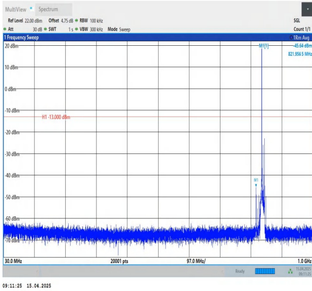
Band26(824-849)-10MHz-QPSK-26990-1RB#0-30~1000-PASS
