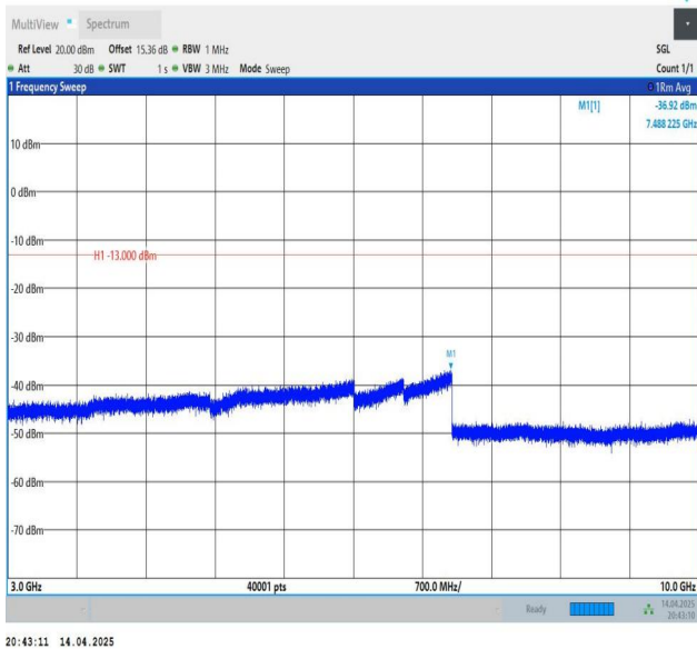
Band26(824-849)-10MHz-QPSK-26990-1RB#0-3000~10000-PAS
