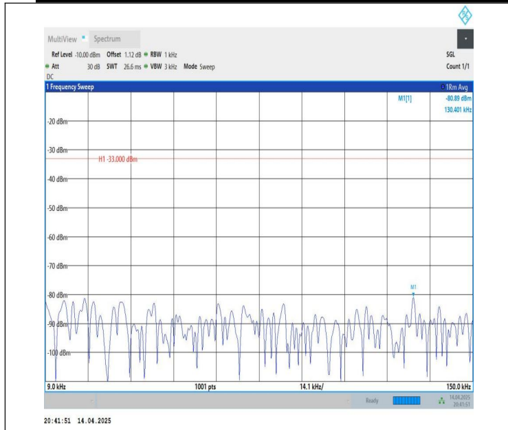
Band26(824-849)-10MHz-QPSK-26915-1RB#0-0.009~0.15-PASS
