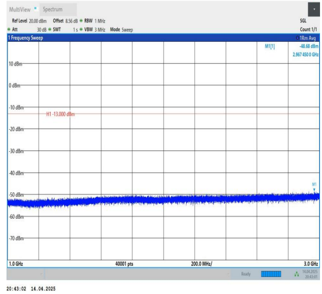
Band26(824-849)-10MHz-QPSK-26990-1RB#0-1000~3000-PASS
