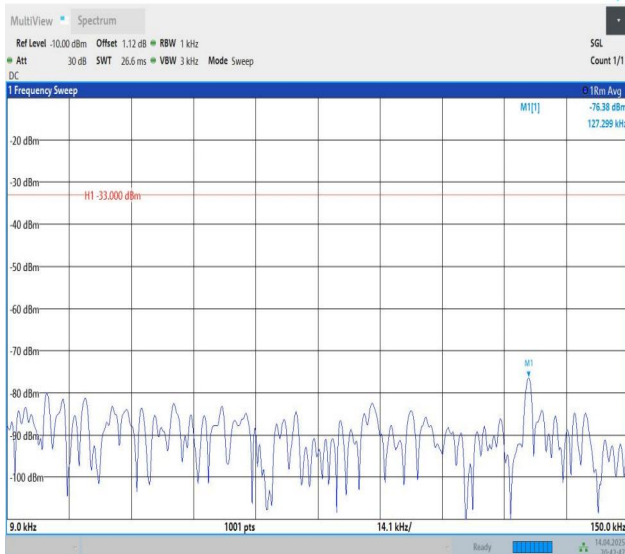
Band26(824-849)-10MHz-QPSK-26990-1RB#0-0.009~0.15-PASS
