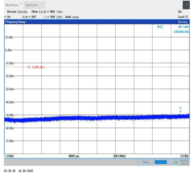
Band26(824-849)-3MHz-QPSK-26805-1RB#0-1000~3000-PASS
