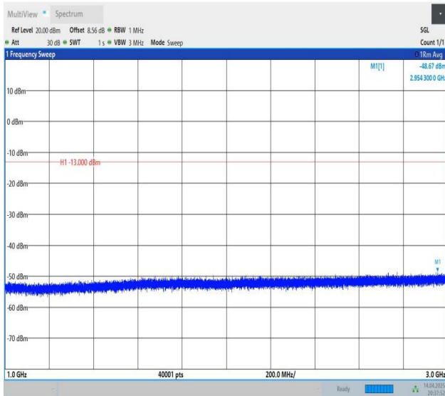
Band26(824-849)-3MHz-QPSK-27025-1RB#14-1000~3000-PASS
