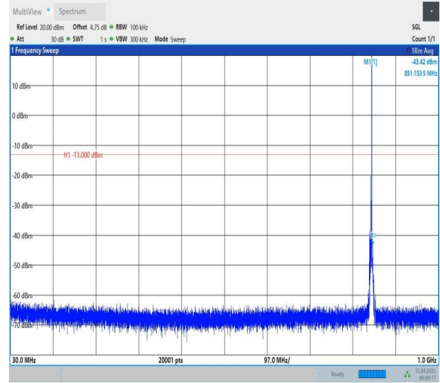
Band26(824-849)-3MHz-QPSK-27025-1RB#14-30~1000-PASS
