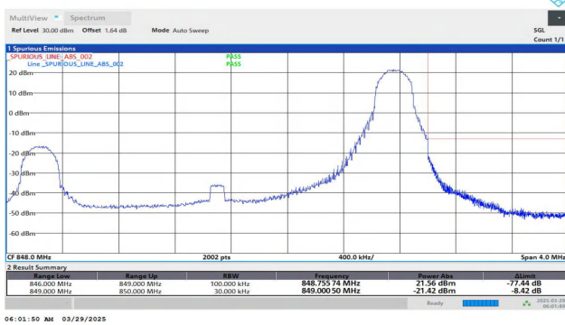
Band26(824-849)-3MHz-QPSK-27025-1RB#14-PASS
