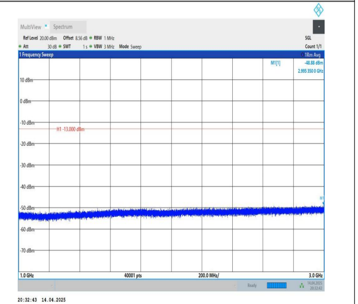
Band26(824-849)-1.4MHz-QPSK-26797-1RB#0-1000~3000-PASS
