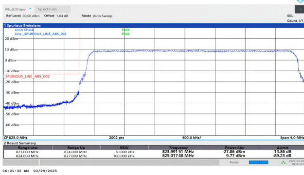
Band26(824-849)-3MHz-QPSK-26805-15RB#0-PASS
