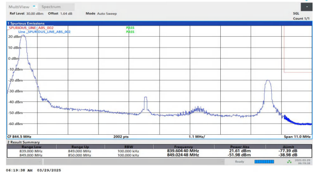
Band26(824-849)-10MHz-QPSK-26990-1RB#0-PASS
