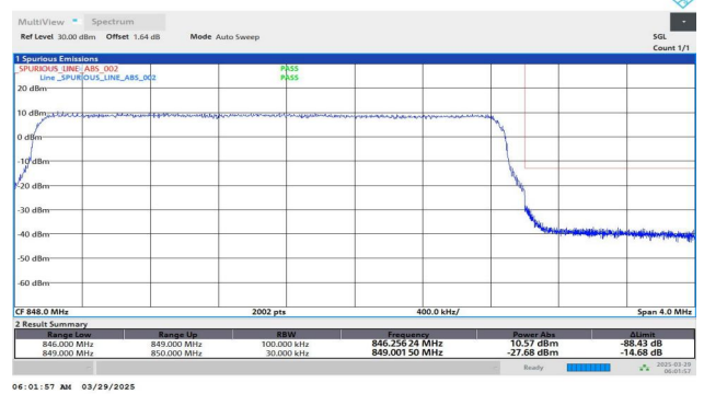
Band26(824-849)-3MHz-QPSK-27025-15RB#0-PASS
