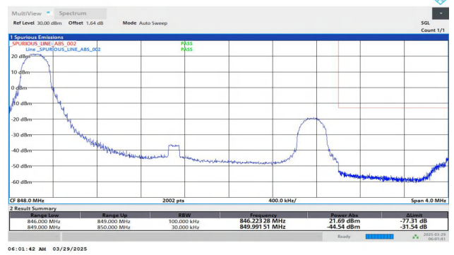
Band26(824-849)-3MHz-QPSK-27025-1RB#0-PASS
