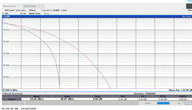
Band26(824-849)-3MHz-QPSK-26915-15RB#0-PASS
