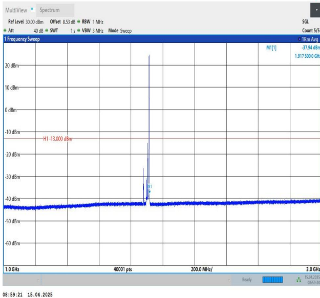
Band25-20MHz-QPSK-26590-1RB#99-1000~3000-PASS
