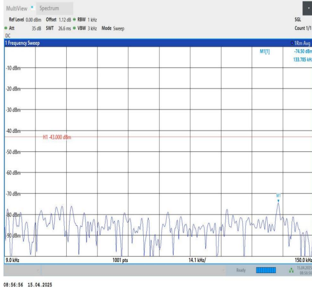
Band25-20MHz-QPSK-26365-1RB#0-0.009~0.15-PASS
