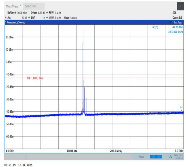
Band25-20MHz-QPSK-26365-1RB#0-1000~3000-PASS
