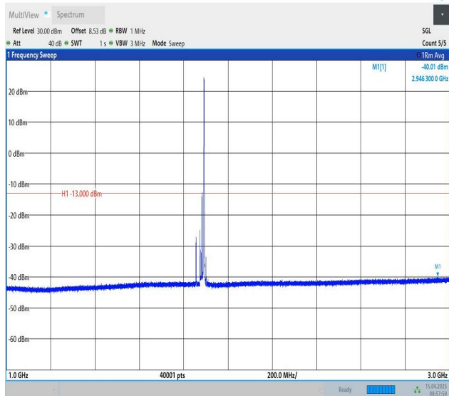
Band25-20MHz-QPSK-26365-1RB#99-1000~3000-PASS
