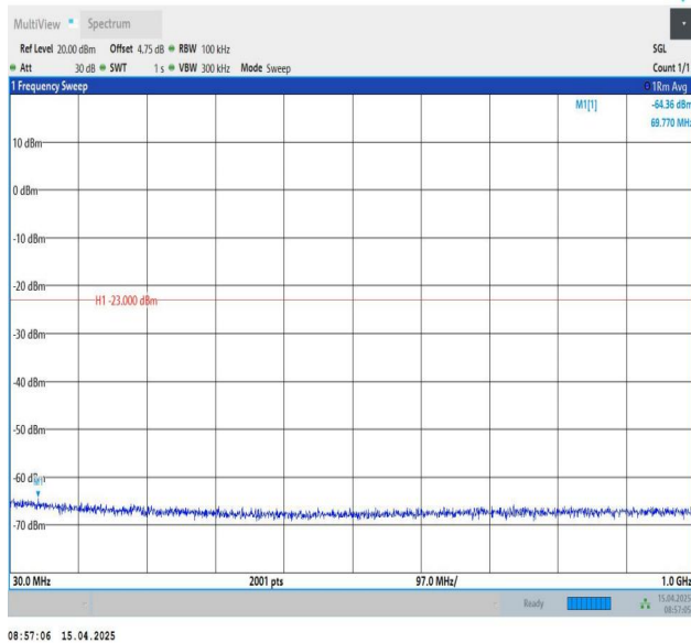
Band25-20MHz-QPSK-26365-1RB#0-30~1000-PASS
