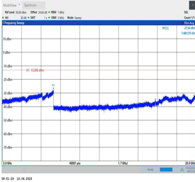
Band25-15MHz-QPSK-26115-1RB#0-3000~20000-PASS
