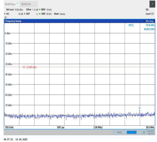
Band25-20MHz-QPSK-26365-1RB#0-0.15~30-PASS
