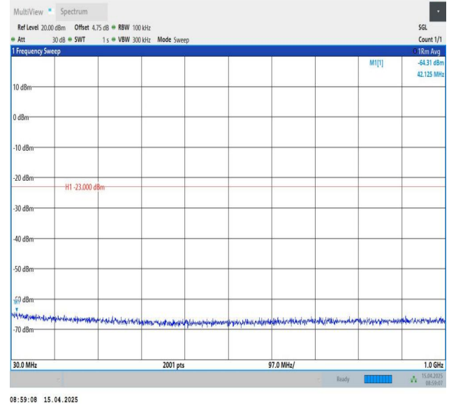
Band25-20MHz-QPSK-26590-1RB#99-30~1000-PASS
