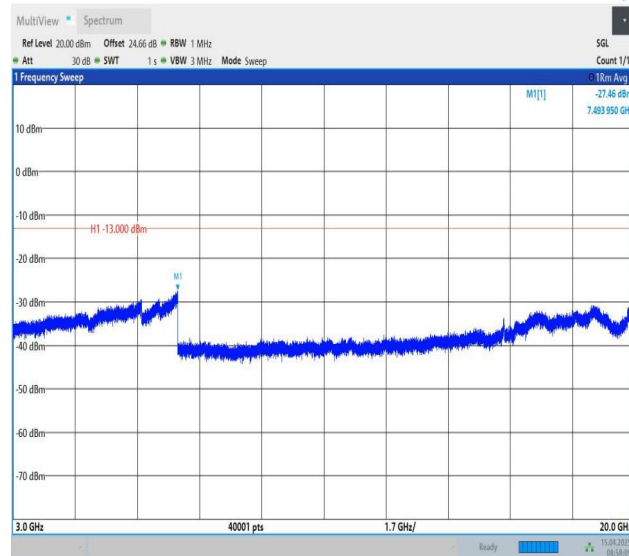
Band25-20MHz-QPSK-26365-1RB#99-3000~20000-PASS
