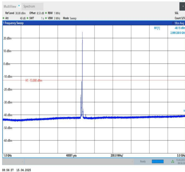
Band25-20MHz-QPSK-26140-1RB#99-1000~3000-PASS
