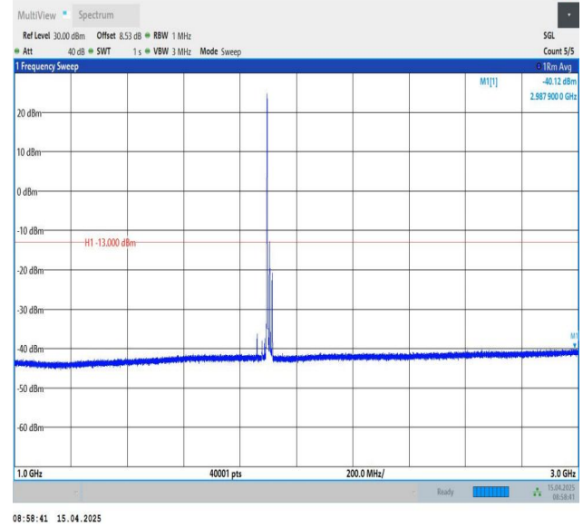
Band25-20MHz-QPSK-26590-1RB#0-1000~3000-PASS
