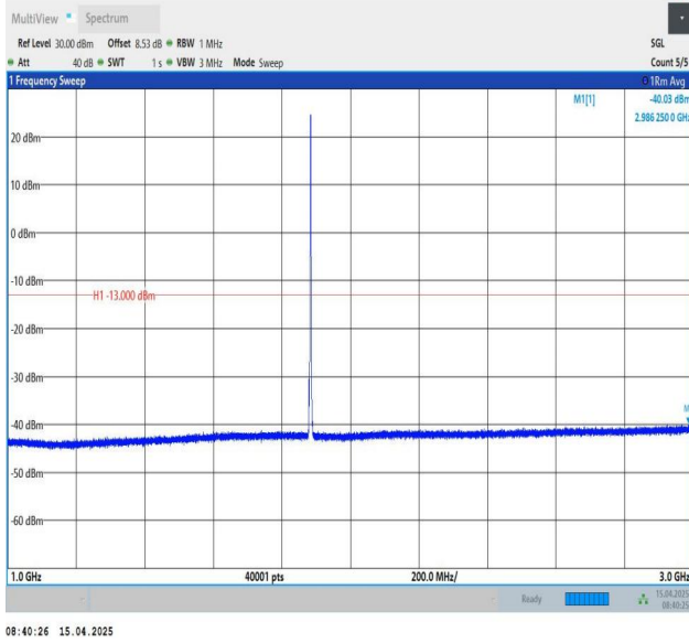
Band25-3MHz-QPSK-26365-1RB#14-1000~3000-PASS
