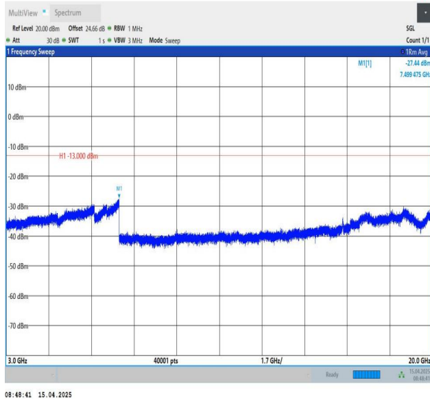
Band25-10MHz-QPSK-26365-1RB#0-3000~20000-PASS
