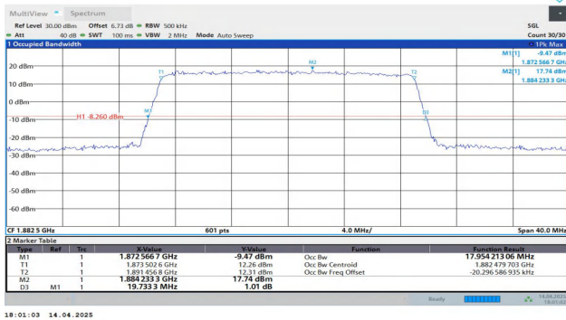
Band25-20MHz-QPSK-26365-100RB#0-PASS
