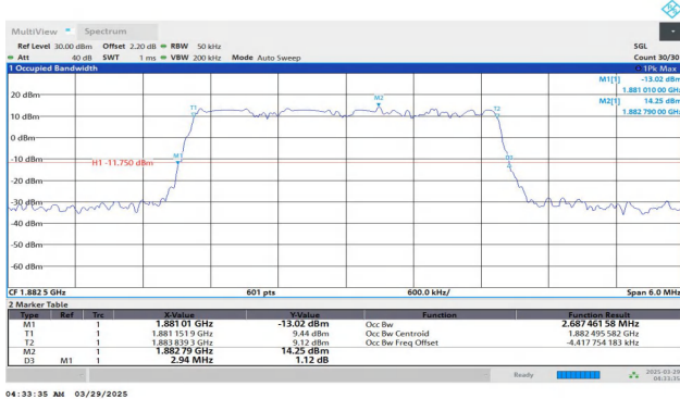
Band25-3MHz-QPSK-26365-15RB#0-PASS
