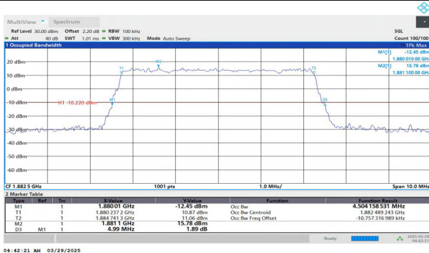
Band25-5MHz-QPSK-26365-25RB#0-PASS
