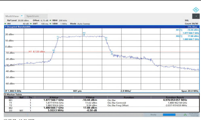
Band25-10MHz-16QAM-26365-27RB#0-PASS
