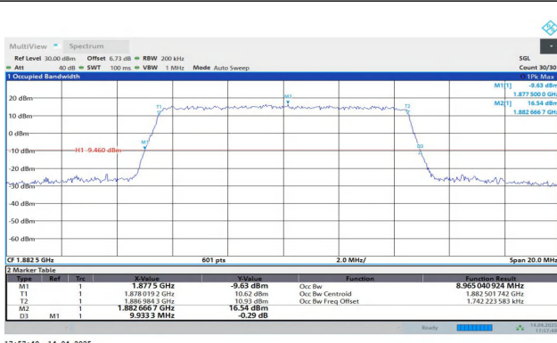
Band25-10MHz-QPSK-26365-50RB#0-PASS
