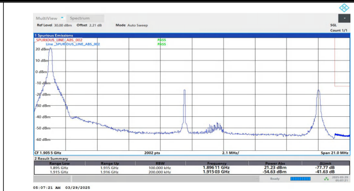
Band25-20MHz-QPSK-26590-1RB#0-PASS
