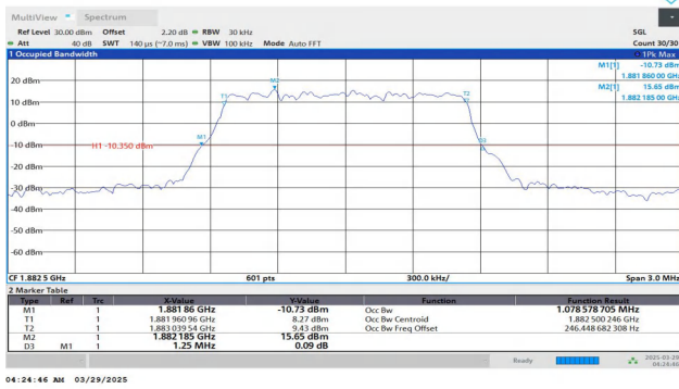
Band25-1.4MHz-QPSK-26365-6RB#0-PASS
