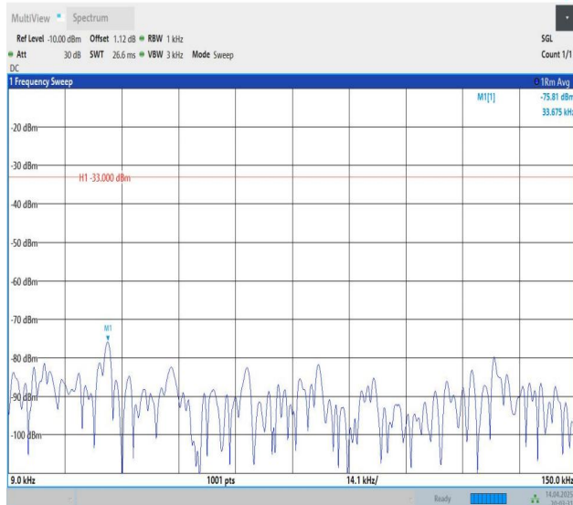
Band5-3MHz-QPSK-20635-1RB#0-0.009~0.15-PASS
