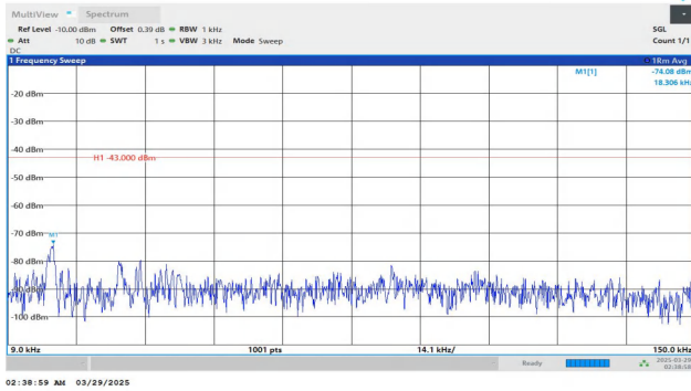
Band4-20MHz-QPSK-20175-1RB#0-0.009~0.15-PASS
