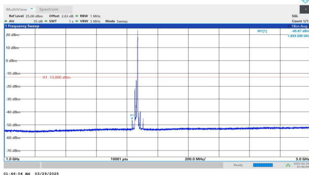
Band2-20MHz-QPSK-18700-1RB#99-1000~3000-PASS
