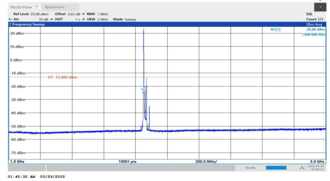
Band2-20MHz-QPSK-18700-1RB#0-1000~3000-PASS
