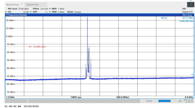
Band2-20MHz-QPSK-18900-1RB#0-1000~3000-PASS
