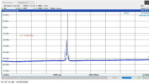
Band2-20MHz-QPSK-18900-1RB#99-1000~3000-PASS
