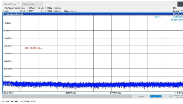
Band2-20MHz-QPSK-18700-1RB#0-30~1000-PASS
