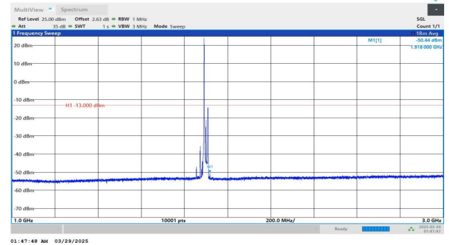
Band2-20MHz-QPSK-19100-1RB#0-1000~3000-PASS
