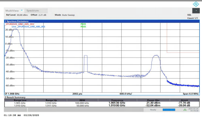
Band2-5MHz-QPSK-19175-1RB#0-PASS
