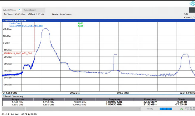
Band2-5MHz-QPSK-18625-1RB#0-PASS
