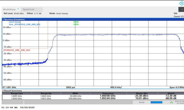
Band2-3MHz-QPSK-18615-15RB#0-PASS
