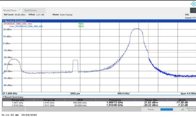
Band2-3MHz-QPSK-19185-1RB#14-PASS
