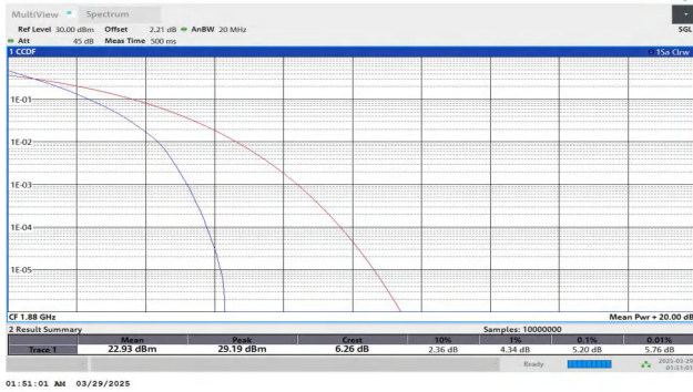
Band2-20MHz-QPSK-18900-100RB#0-PASS
