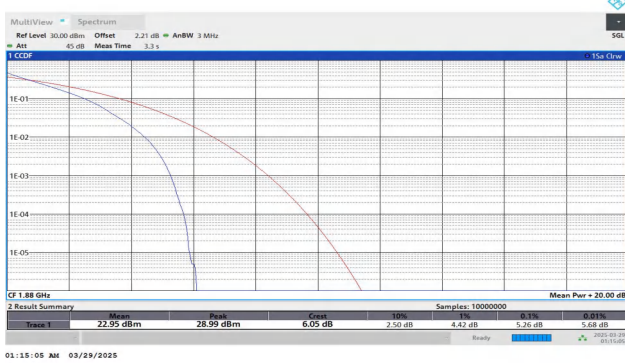
Band2-3MHz-QPSK-18900-15RB#0-PASS
