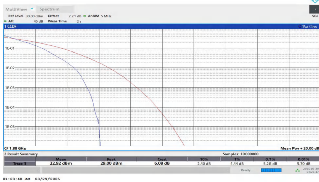
Band2-5MHz-QPSK-18900-25RB#0-PASS
