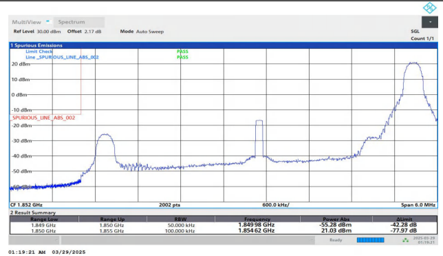
Band2-5MHz-QPSK-18625-1RB#24-PASS
