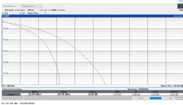
Band2-10MHz-QPSK-18900-50RB#0-PASS
