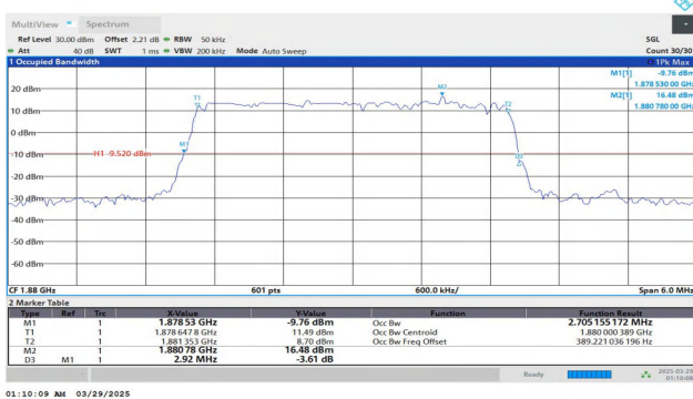
Band2-3MHz-QPSK-18900-15RB#0-PASS
