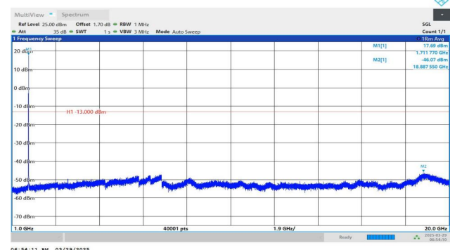
Band4-1312-4-1000~20000MHz-PASS
