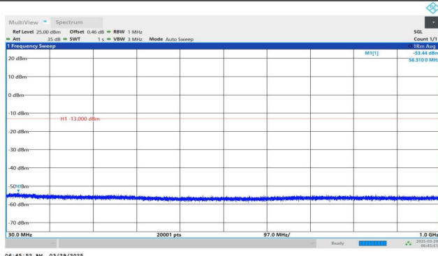
Band4-1513-2-30~1000MHz-PASS
