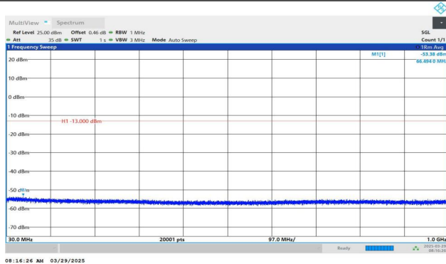
Band4-1312-4-30~1000MHz-PASS
