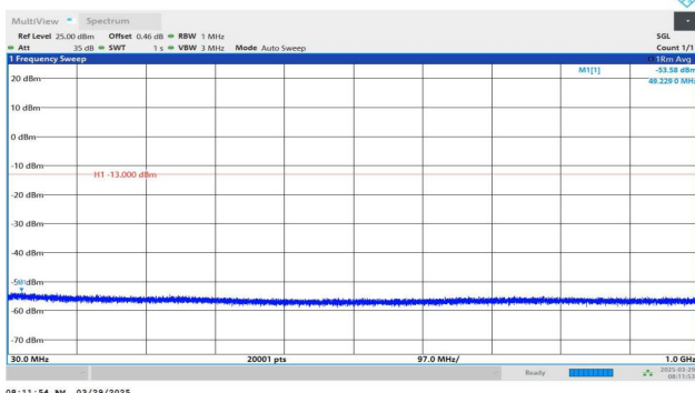
Band4-1513-2-30~1000MHz-PASS
