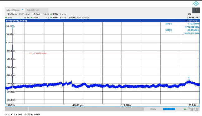
Band4-1312-4-1000~20000MHz-PASS
