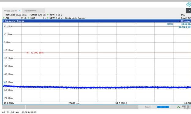
Band4-1312-30~1000MHz-PASS
