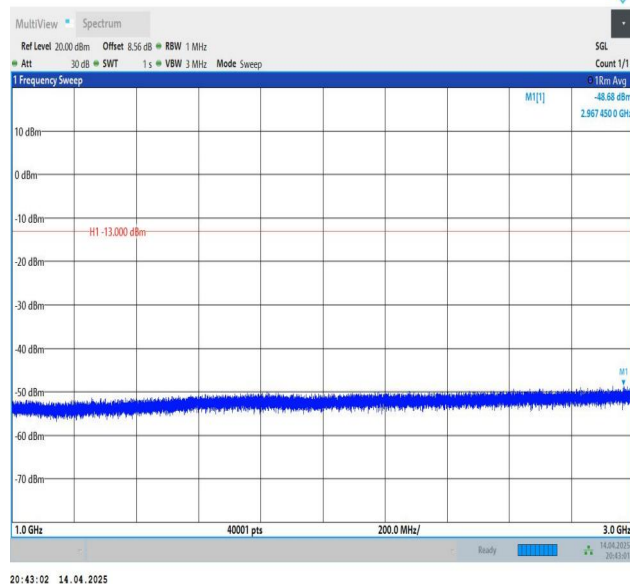
Band26(824-849)-10MHz-QPSK-26990-1RB#0-1000~3000-PASS
