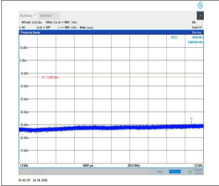
Band26(824-849)-10MHz-QPSK-26990-1RB#49-1000~3000-PAS
