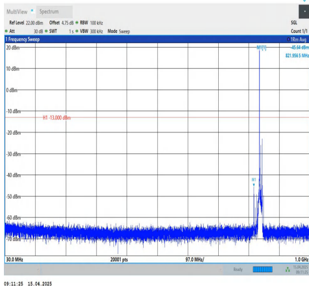
Band26(824-849)-10MHz-QPSK-26990-1RB#0-30~1000-PASS
