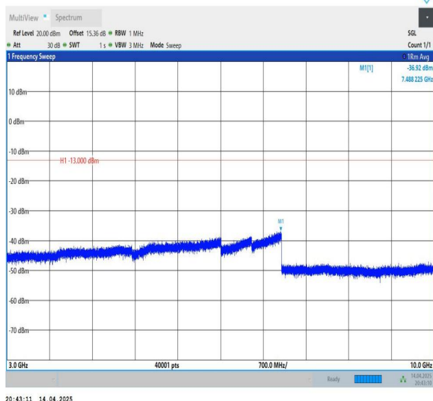
Band26(824-849)-10MHz-QPSK-26990-1RB#0-3000~10000-PAS
