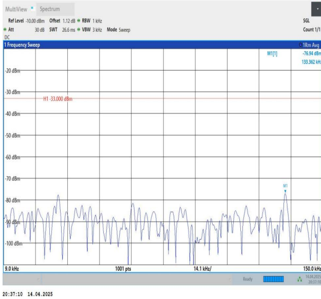
Band26(824-849)-3MHz-QPSK-27025-1RB#0-0.009~0.15-PASS
