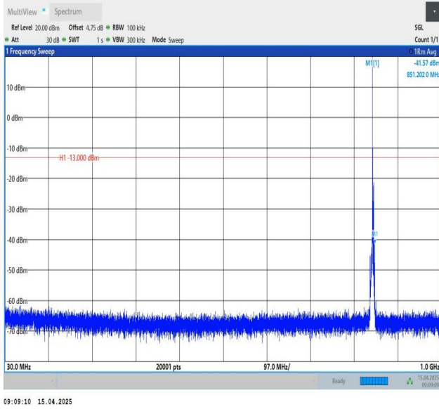
Band26(824-849)-3MHz-QPSK-27025-1RB#0-30~1000-PASS
