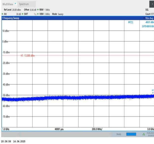
Band26(824-849)-3MHz-QPSK-26915-1RB#14-1000~3000-PASS
