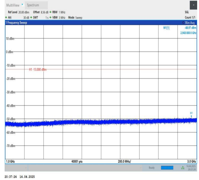
Band26(824-849)-3MHz-QPSK-27025-1RB#0-1000~3000-PASS
