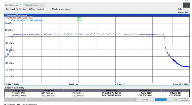
Band26(824-849)-10MHz-QPSK-26990-50RB#0-PASS
