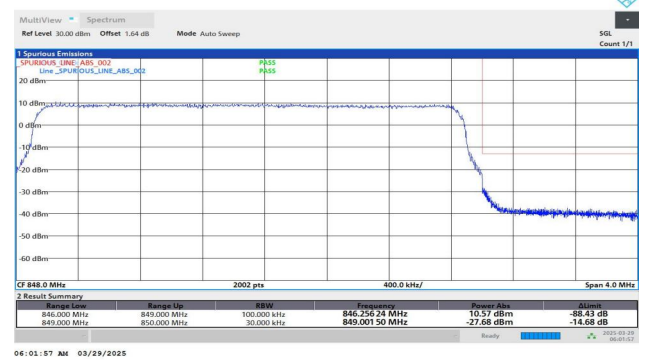
Band26(824-849)-3MHz-QPSK-27025-15RB#0-PASS
