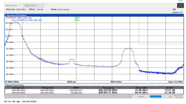
Band26(824-849)-3MHz-QPSK-27025-1RB#0-PASS
