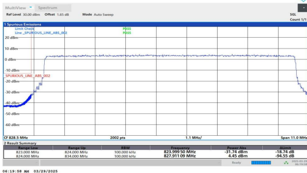
Band26(824-849)-10MHz-QPSK-26840-50RB#0-PASS
