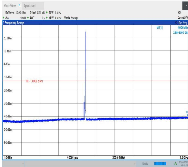
Band25-10MHz-QPSK-26365-1RB#49-1000~3000-PASS
