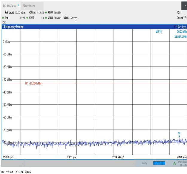
Band25-20MHz-QPSK-26365-1RB#99-0.15~30-PASS
