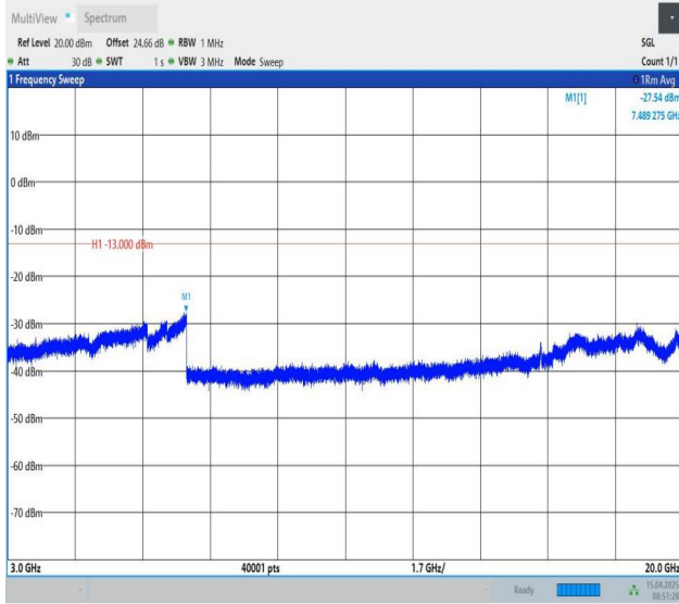
Band25-15MHz-QPSK-26115-1RB#0-3000~20000-PASS
