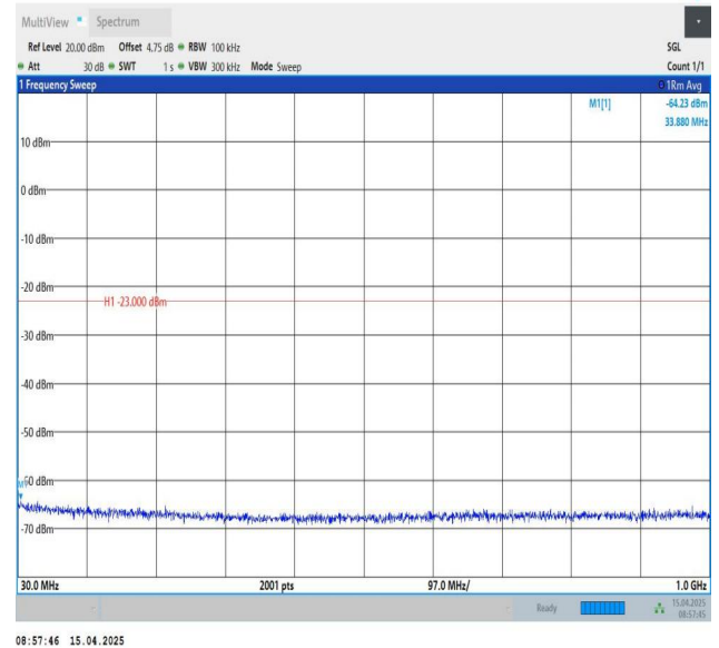
Band25-20MHz-QPSK-26365-1RB#99-30~1000-PASS
