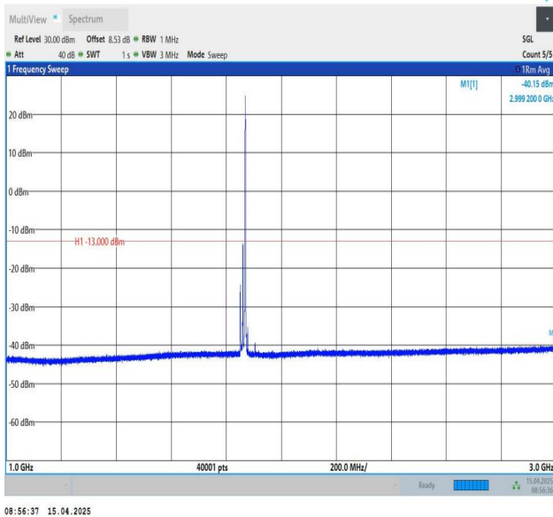
Band25-20MHz-QPSK-26140-1RB#99-1000~3000-PASS
