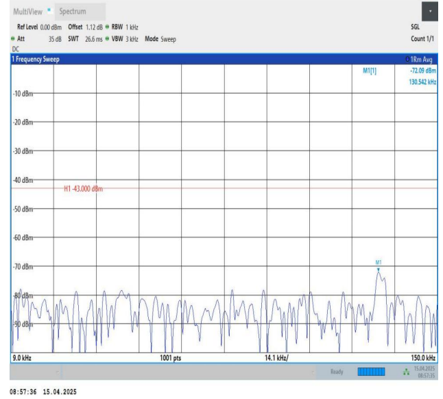
Band25-20MHz-QPSK-26365-1RB#99-0.009~0.15-PASS
