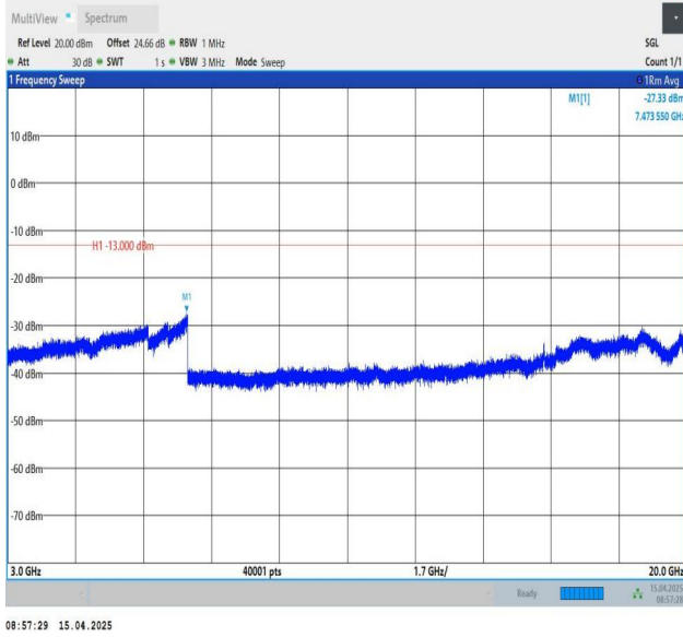
Band25-20MHz-QPSK-26365-1RB#0-3000~20000-PASS
