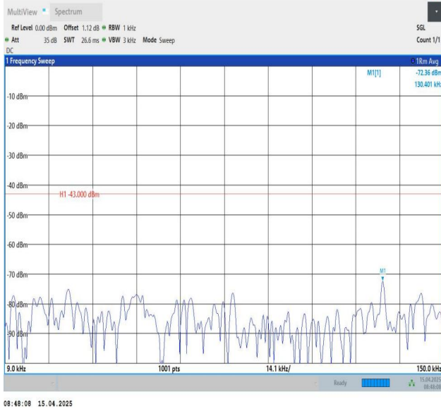
Band25-10MHz-QPSK-26365-1RB#0-0.009~0.15-PASS
