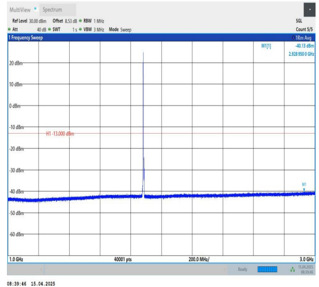
Band25-3MHz-QPSK-26365-1RB#0-1000~3000-PASS
