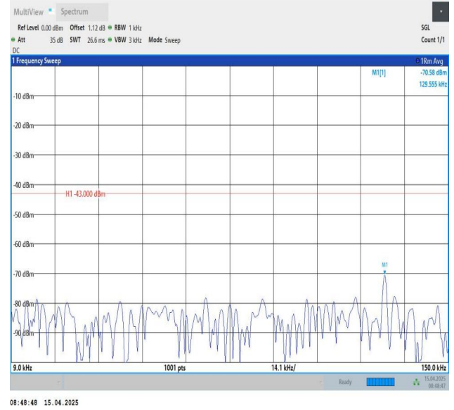
Band25-10MHz-QPSK-26365-1RB#49-0.009~0.15-PASS
