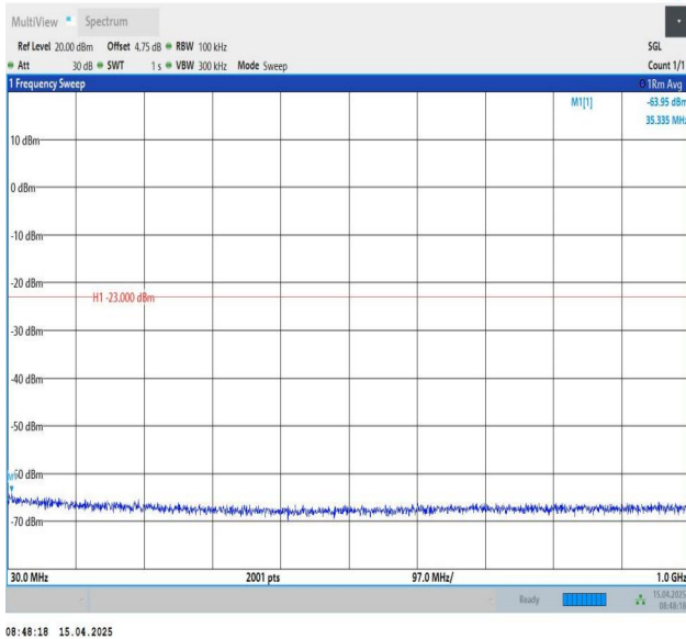
Band25-10MHz-QPSK-26365-1RB#0-30~1000-PASS
