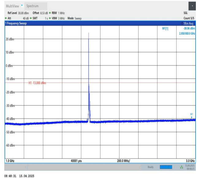
Band25-10MHz-QPSK-26365-1RB#0-1000~3000-PASS
