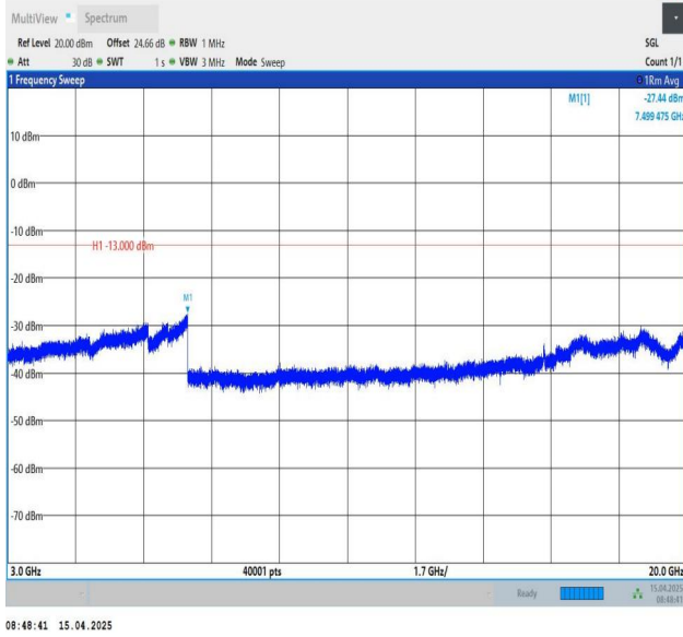
Band25-10MHz-QPSK-26365-1RB#0-3000~20000-PASS
