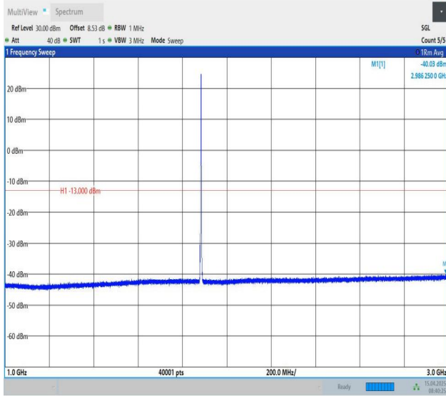
Band25-3MHz-QPSK-26365-1RB#14-1000~3000-PASS
