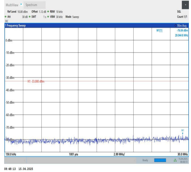
Band25-10MHz-QPSK-26365-1RB#0-0.15~30-PASS
