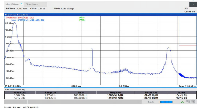
Band25-10MHz-QPSK-26640-1RB#0-PASS
