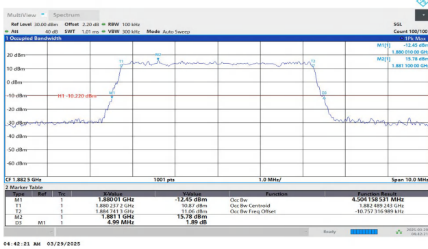
Band25-5MHz-QPSK-26365-25RB#0-PASS
