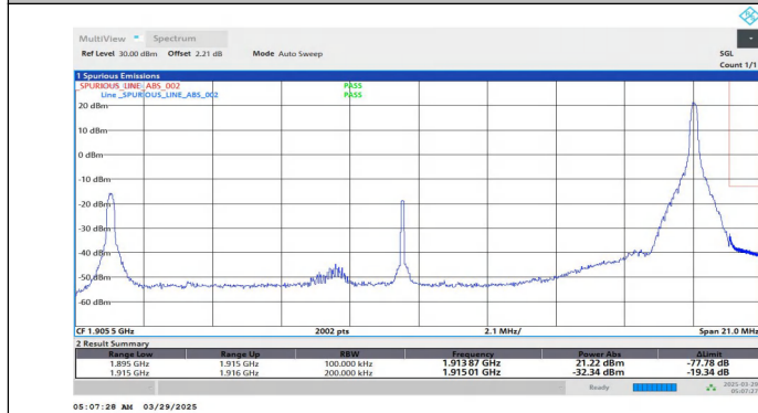
Band25-20MHz-QPSK-26590-1RB#99-PASS
