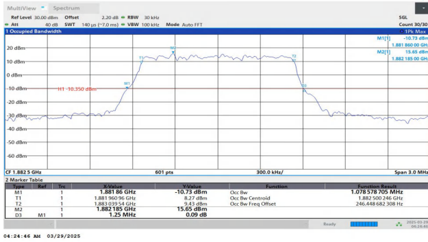
Band25-1.4MHz-QPSK-26365-6RB#0-PASS
