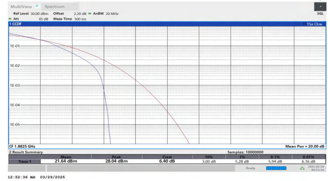
Band25-20MHz-16QAM-26365-27RB#0-PASS
