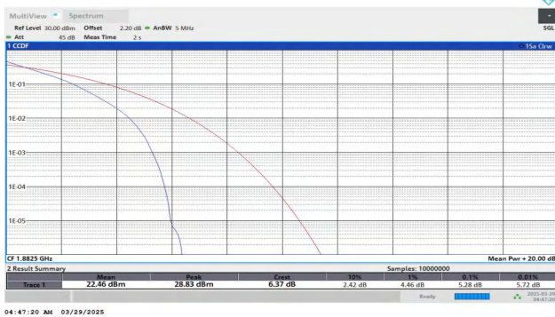
Band25-5MHz-QPSK-26365-25RB#0-PASS
