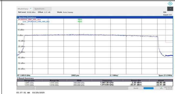
Band25-20MHz-QPSK-26590-100RB#0-PASS
