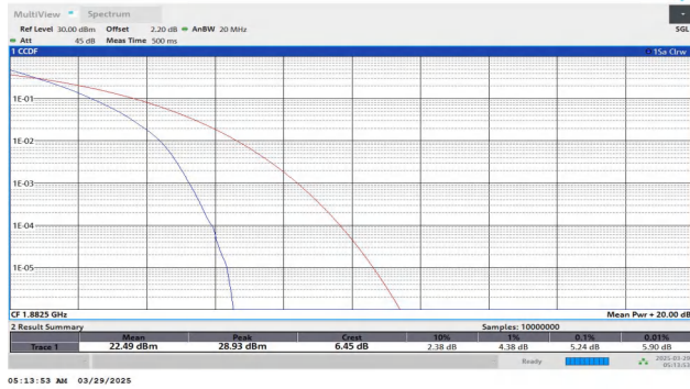
Band25-20MHz-QPSK-26365-100RB#0-PASS
