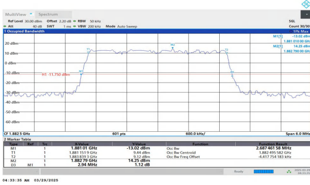
Band25-3MHz-QPSK-26365-15RB#0-PASS
