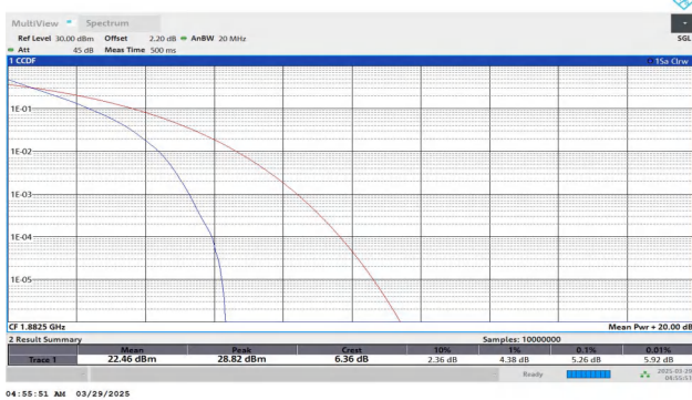
Band25-10MHz-QPSK-26365-50RB#0-PASS
