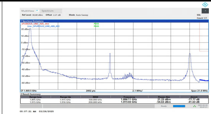
Band25-20MHz-QPSK-26590-1RB#0-PASS
