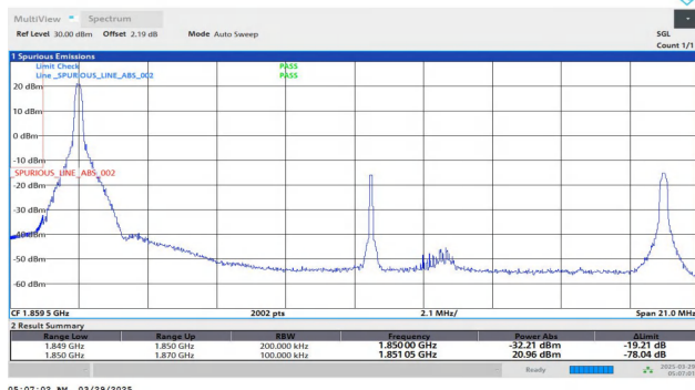
Band25-20MHz-QPSK-26140-1RB#0-PASS
