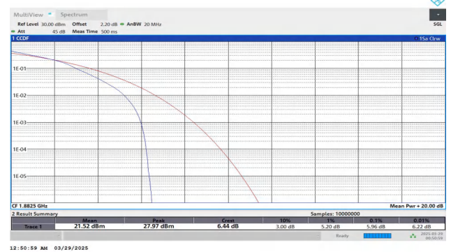
Band25-10MHz-16QAM-26365-27RB#0-PASS
