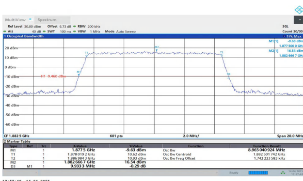
Band25-10MHz-QPSK-26365-50RB#0-PASS
