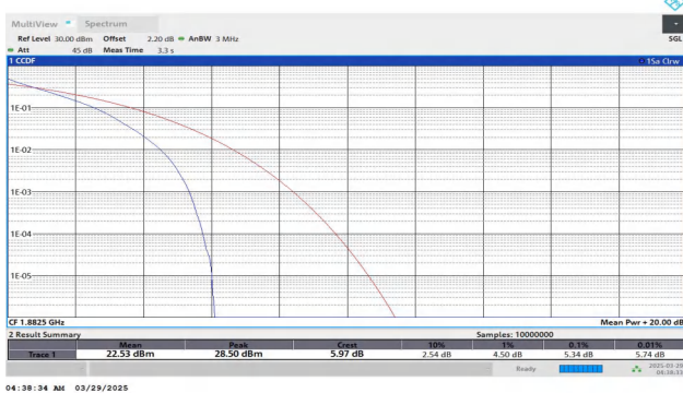
Band25-3MHz-QPSK-26365-15RB#0-PASS
