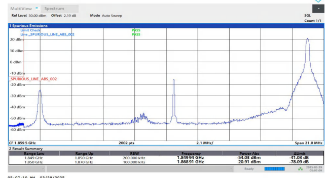
Band25-20MHz-QPSK-26140-1RB#99-PASS
