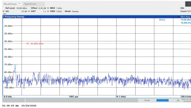
Band4-20MHz-QPSK-20175-1RB#0-0.009~0.15-PASS
