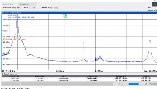
Band4-20MHz-QPSK-20050-1RB#0-PASS
