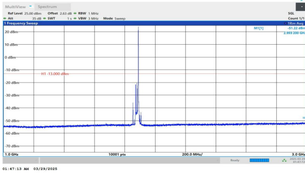
Band2-20MHz-QPSK-18900-1RB#99-1000~3000-PASS
