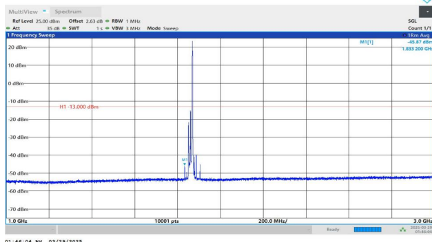
Band2-20MHz-QPSK-18700-1RB#99-1000~3000-PASS
