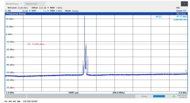
Band2-20MHz-QPSK-18900-1RB#0-1000~3000-PASS
