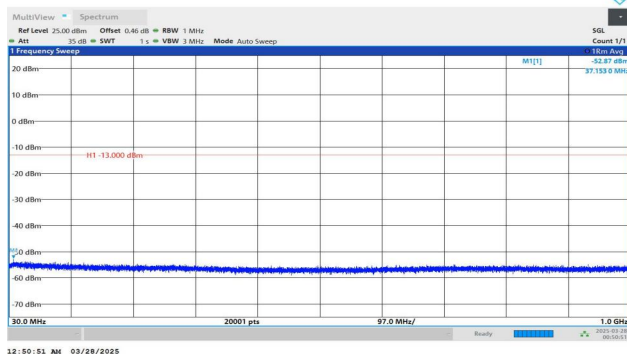
Band2-9538-2-30~1000MHz-PASS
