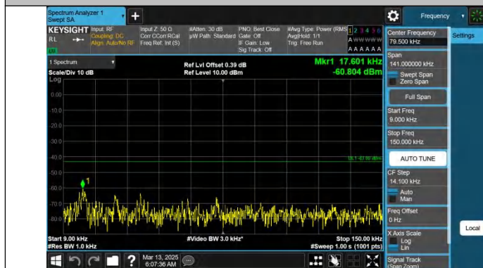
Band66-20MHz-QPSK-132572-1RB#0-0.009~0.15-PASS
