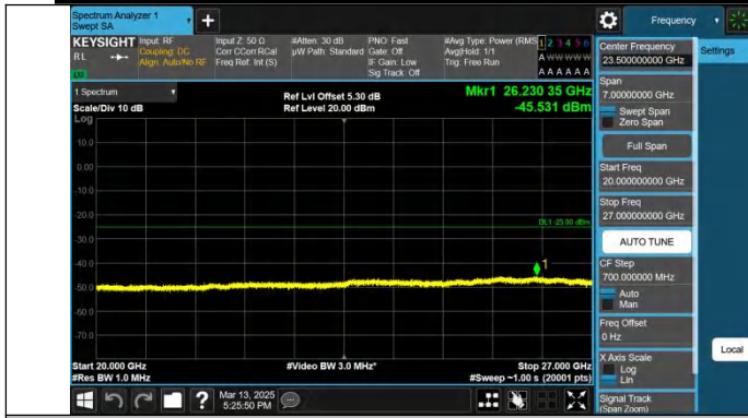
Band41-15MHz-QPSK-39725-1RB#0-20000~27000-PASS
