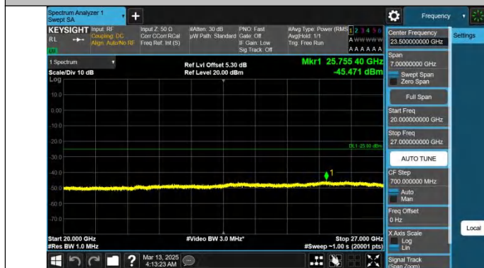
Band38-20MHz-QPSK-38150-1RB#0-20000~27000-PASS
