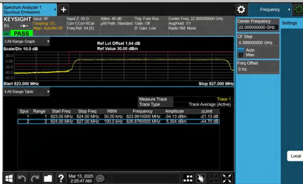
Band26(824-849)-3MHz-QPSK-26805-15RB#0-PASS
