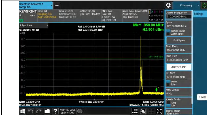
Band26(824-849)-10MHz-QPSK-26990-1RB#0-30~1000-PASS
