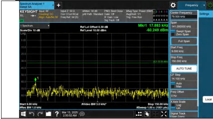
Band26(824-849)-10MHz-QPSK-26990-1RB#0-0.009~0.15-PASS
