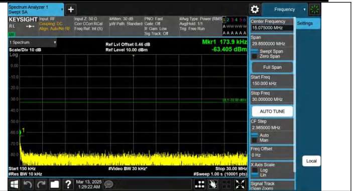
Band25-20MHz-QPSK-26365-1RB#0-0.15~30-PASS
