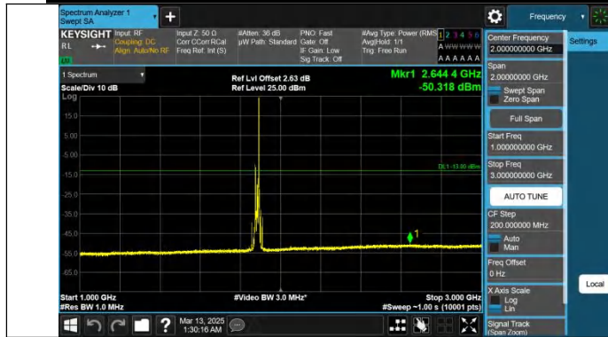
Band25-20MHz-QPSK-26365-1RB#99-1000~3000-PASS
