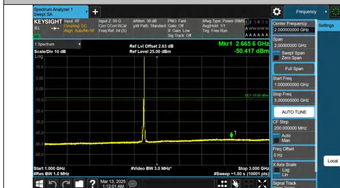
Band25-10MHz-QPSK-26365-1RB#49-1000~3000-PASS
