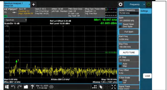
Band25-10MHz-QPSK-26365-1RB#49-0.009~0.15-PASS
