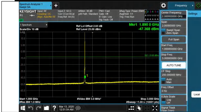
Band25-3MHz-QPSK-26365-1RB#14-1000~3000-PASS
