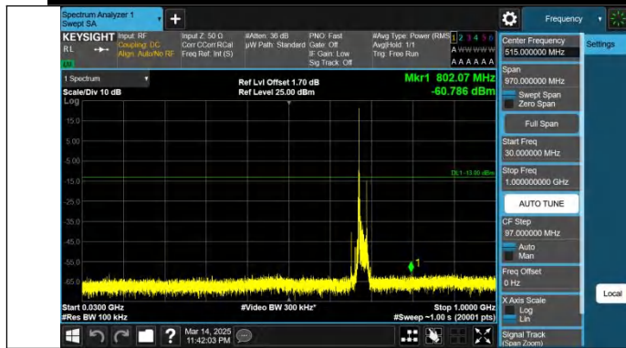
Band71-20MHz-QPSK-133372-1RB#0-30~1000-PASS
