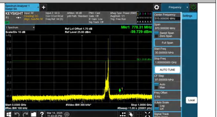
Band71-20MHz-QPSK-133372-1RB#99-30~1000-PASS
