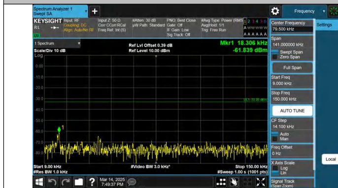
Band5-3MHz-QPSK-20635-1RB#0-0.009~0.15-PASS
