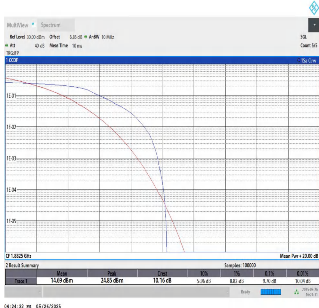
Band25-10MHz-QPSK-26365-PASS
