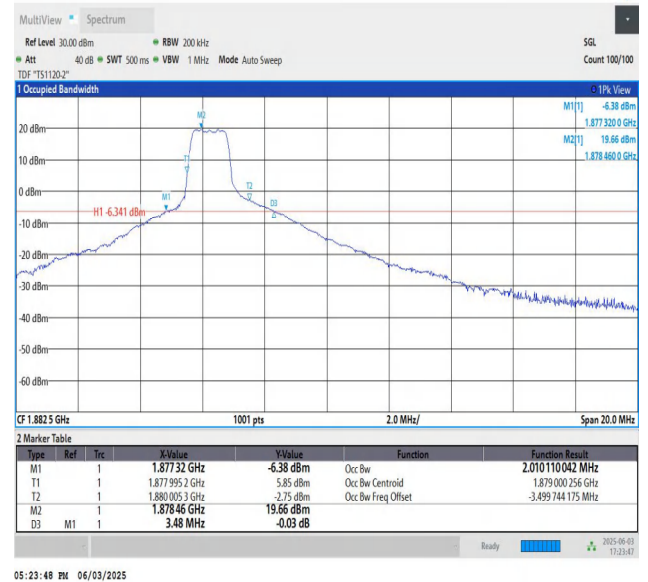
Band25-10MHz-16QAM-26365-PASS
