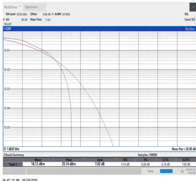
Band25-20MHz-QPSK-26365-PASS
