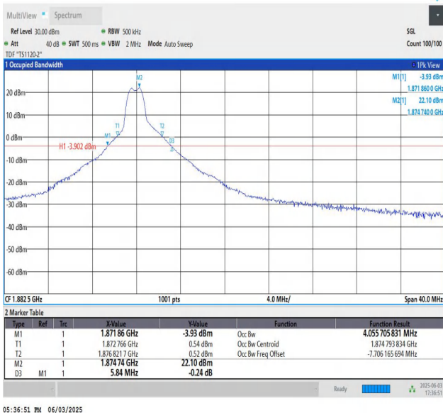
Band25-20MHz-QPSK-26365-PASS
