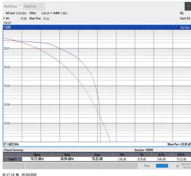
Band25-5MHz-QPSK-26365-PASS
