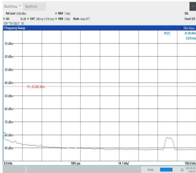
Band25-10MHz-QPSK-26365-PASS
