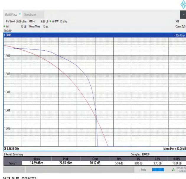
Band25-10MHz-16QAM-26365-PASS
