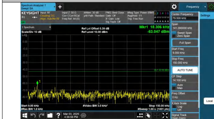
Band25-10MHz-QPSK-26365-1RB#0-0.009~0.15-PASS
