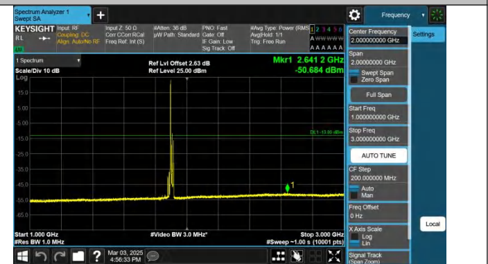
Band25-20MHz-QPSK-26590-1RB#0-1000~3000-PASS
