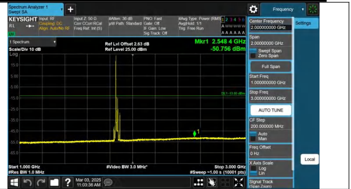
Band2-20MHz-QPSK-18700-1RB#0-1000~3000-PASS
