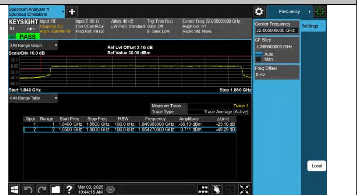
Band2-10MHz-QPSK-18650-50RB#0-PASS
