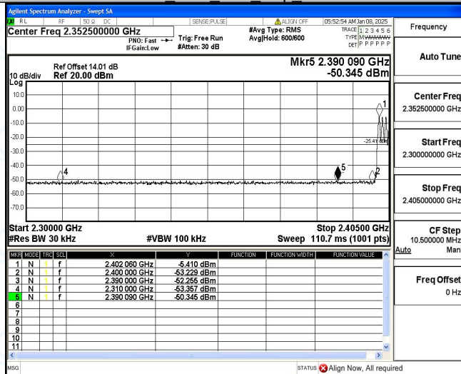
DH5_Ant1_Low_Hop_2402
