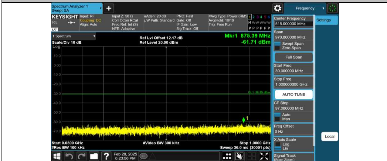
11G-Ant1-2462-30~1000-PASS
