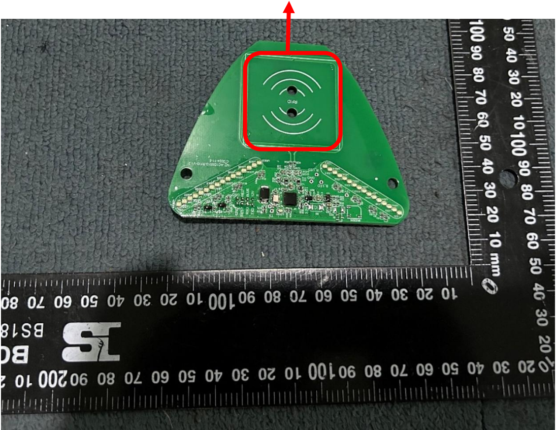
RFID Antenna
