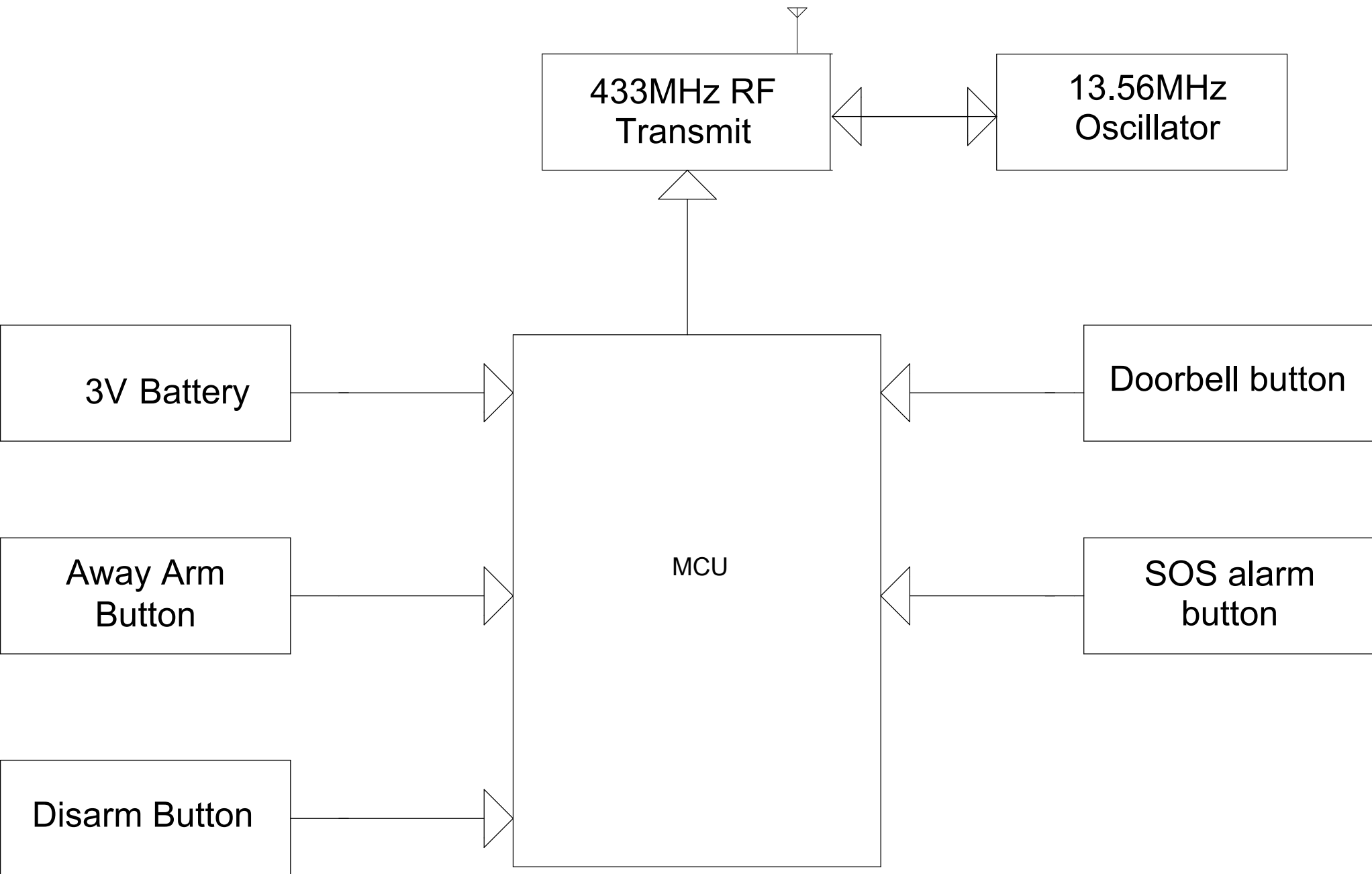
MC-02B方框图 深圳市艾瑞泽电子有限公司 2025-05-27
