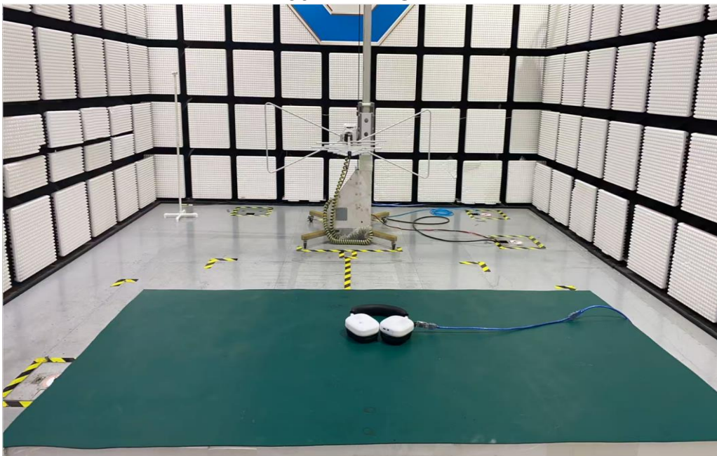
30MHz ~ 1GHz
