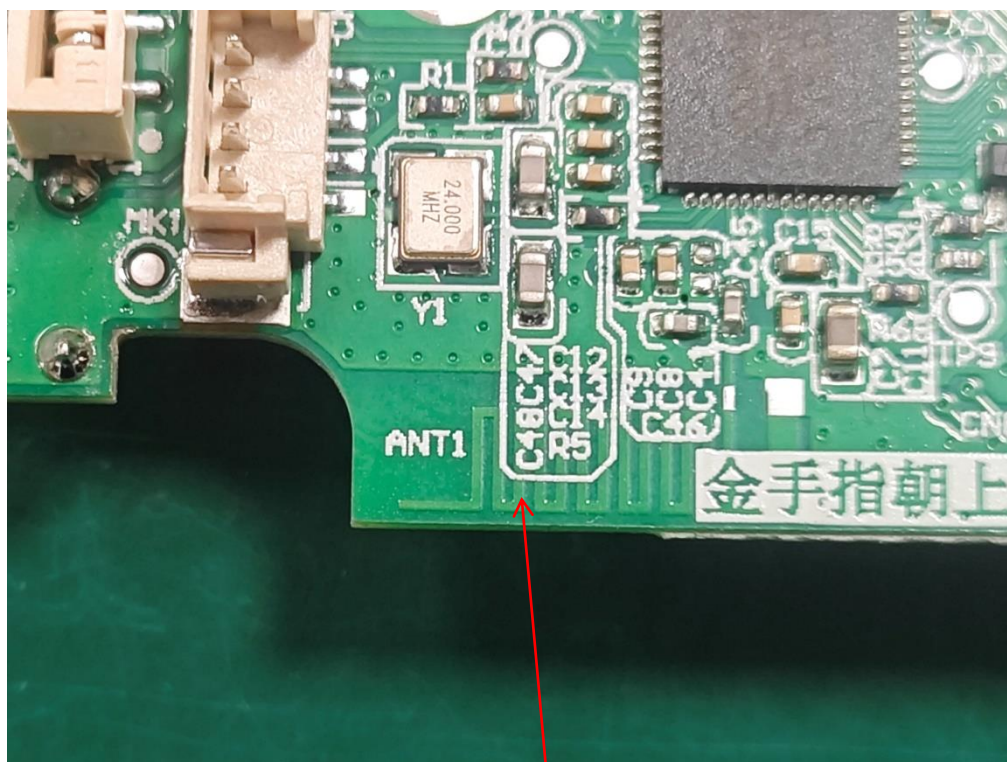
BT and BLE ANT
