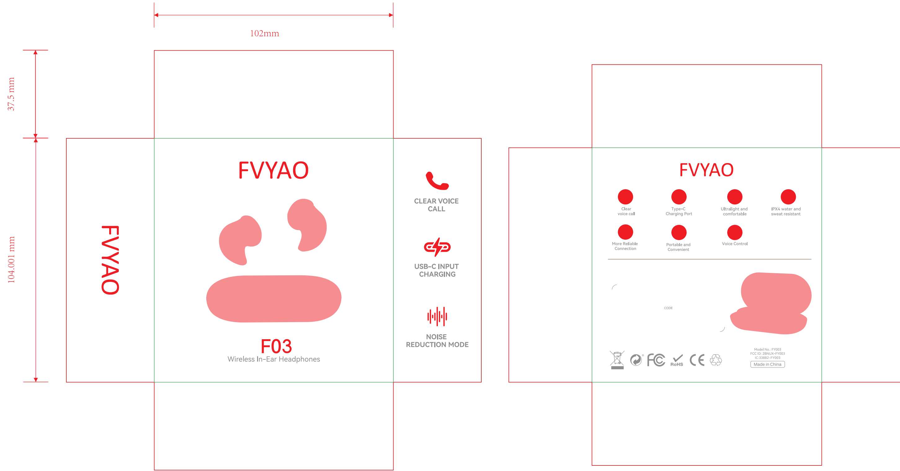
157G双铜+哑胶UV( 红色区域 )+4C+877C印刷+1200G白板104x102x37.5mm
