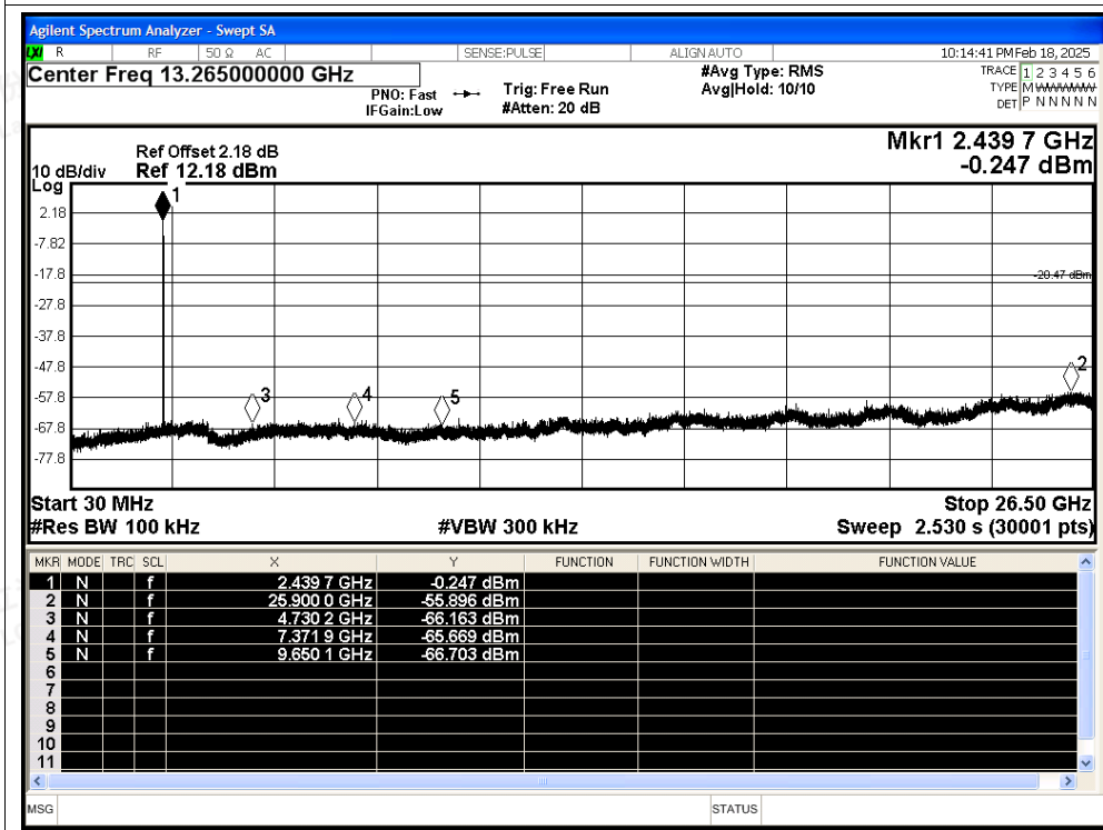
Tx. Spurious NVNT BLE 2M 2440MHz Ant Emission
