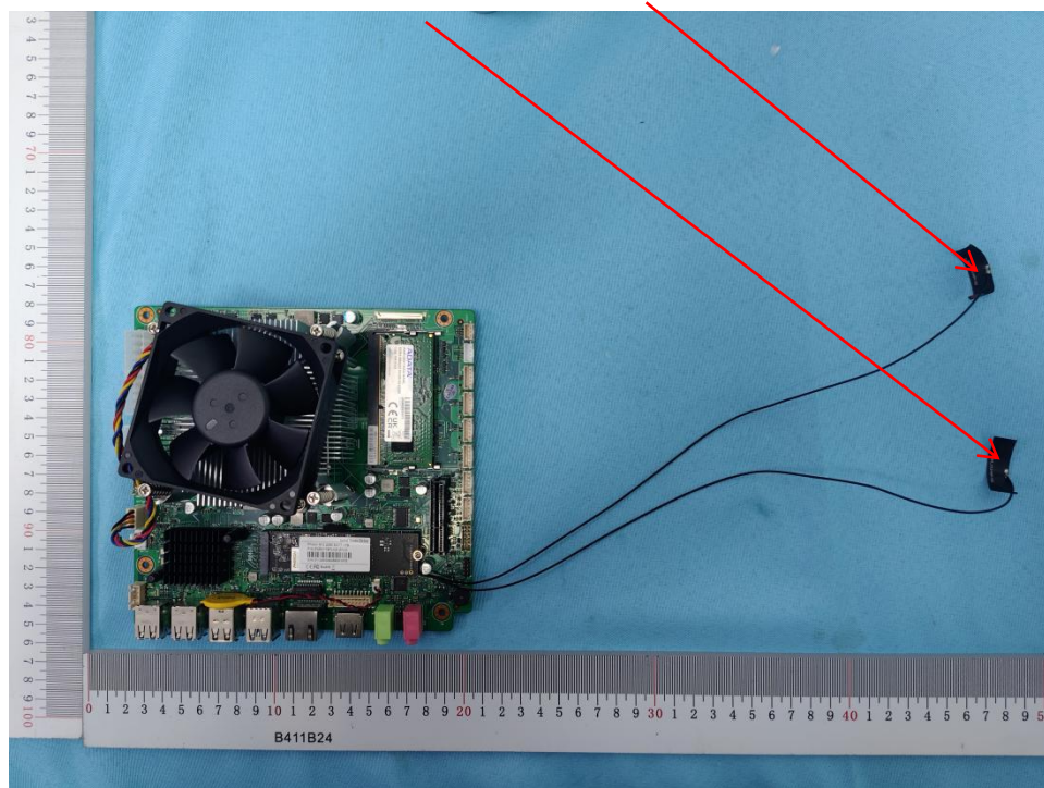
2.4G&5G&BT-ANT1
