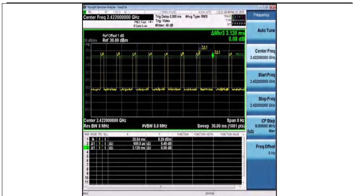
NTNV-11AX40MIMO-Ant1-2422
