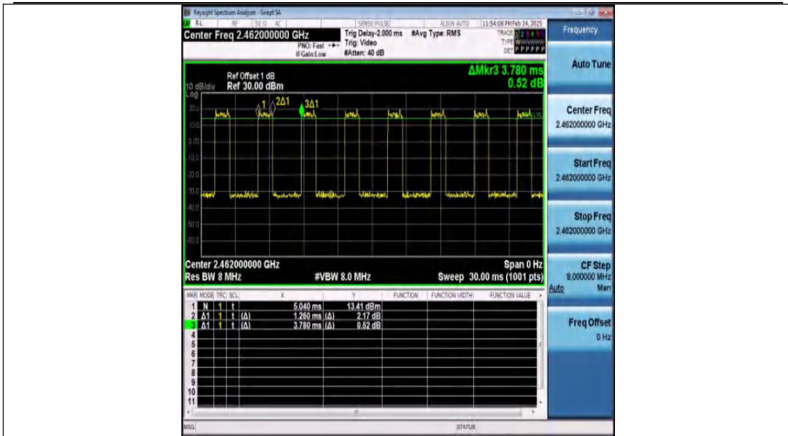
NTNV-11N20MIMO-Ant1-2462
