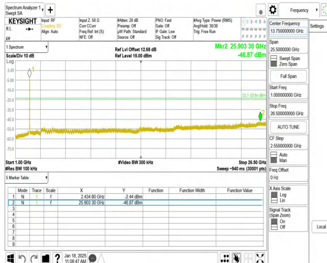
11AX40MIMO_Ant1_2437_1000~26500
