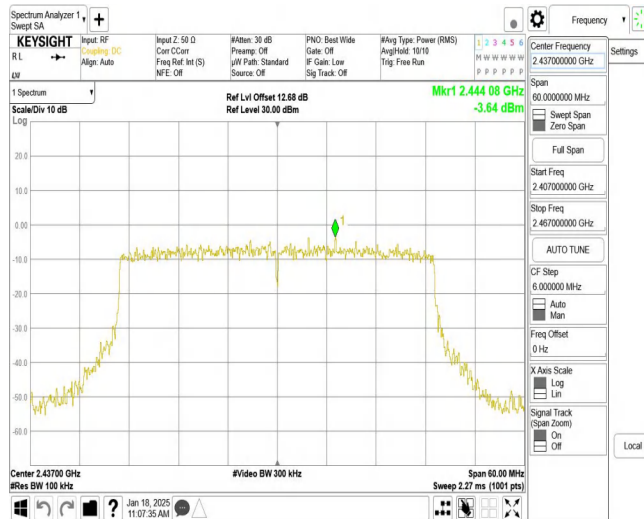
11AX40MIMO_Ant1_2437_0~Reference
