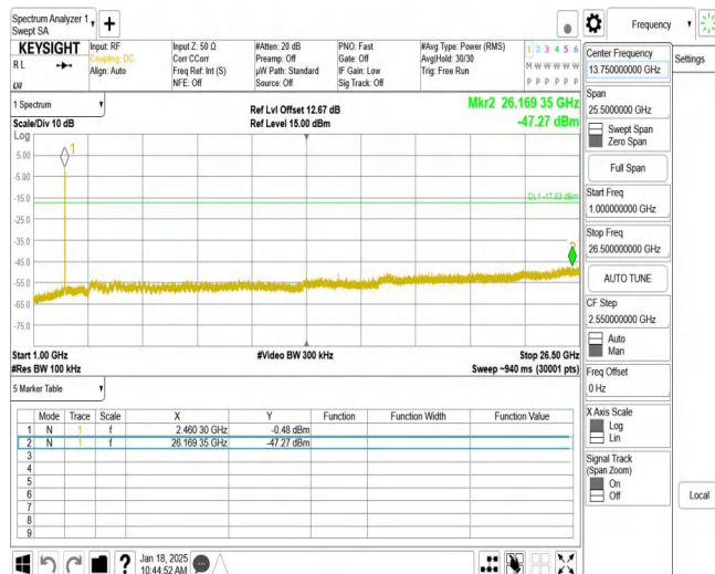
11AX20MIMO_Ant1_2462_1000~26500
