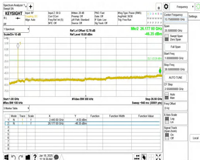
11AX40MIMO_Ant2_2437_1000~26500
