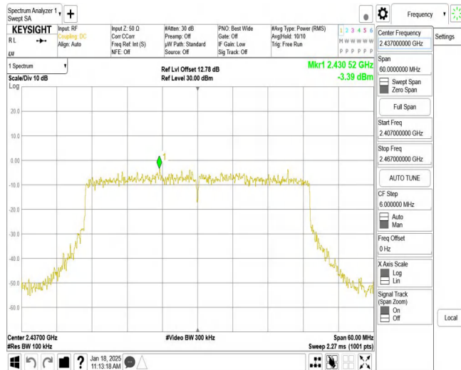
11AX40MIMO_Ant2_2437_0~Reference
