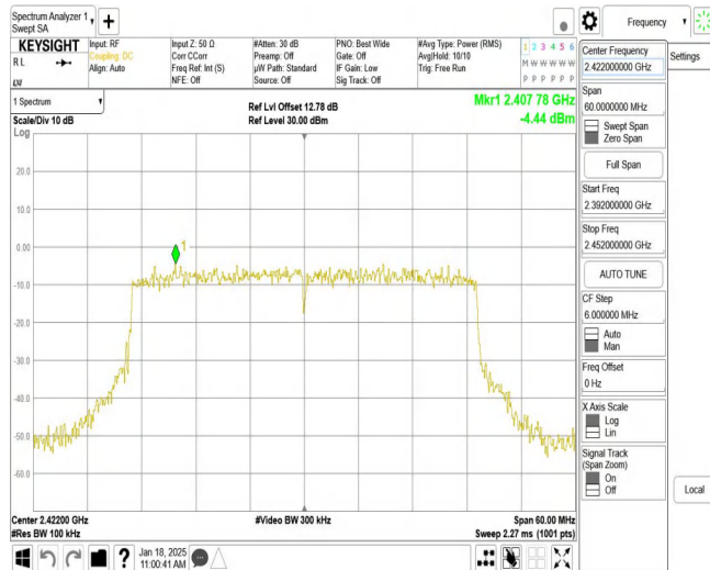
11AX40MIMO_Ant2_2422_0~Reference
