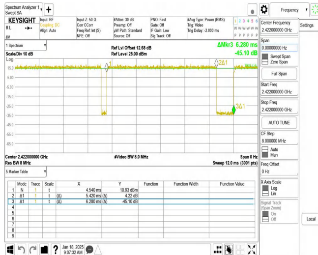
11N40MIMO_Ant1_2422
