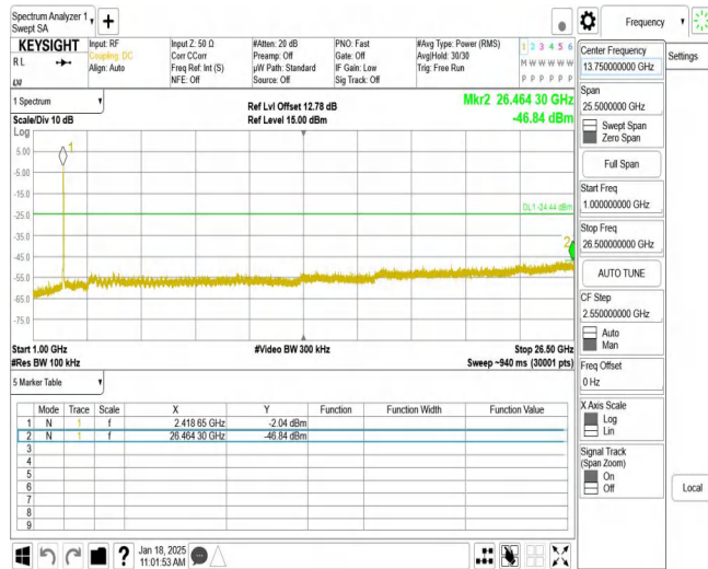
11AX40MIMO_Ant2_2422_1000~26500
