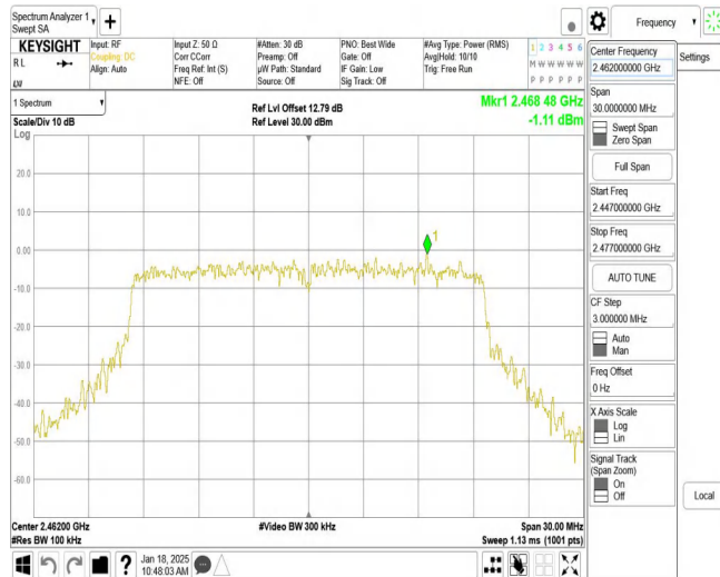
11AX20MIMO_Ant2_2462_0~Reference
