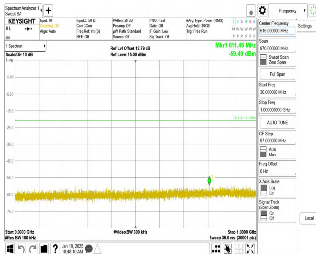
11AX20MIMO_Ant2_2462_30~1000
