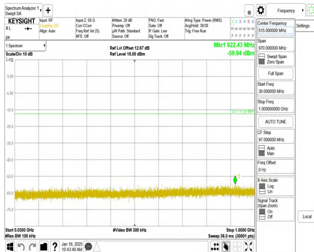
11AX20MIMO_Ant1_2462_30~1000
