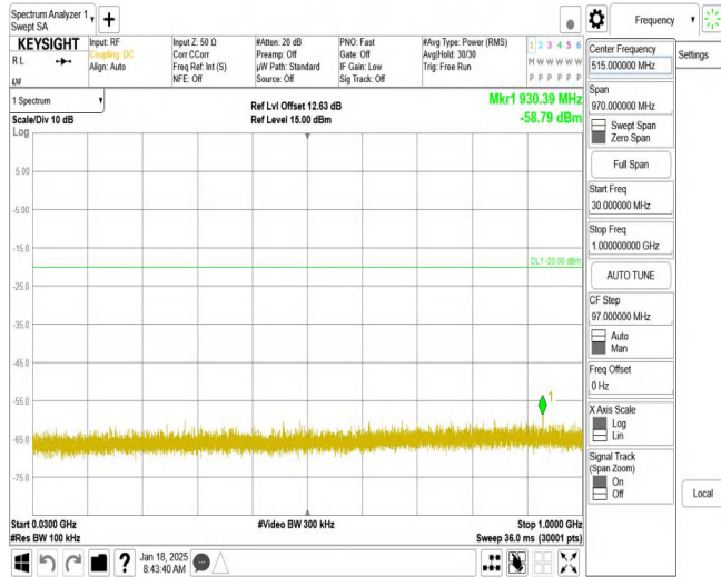
11N20MIMO_Ant1_2412_30~1000
