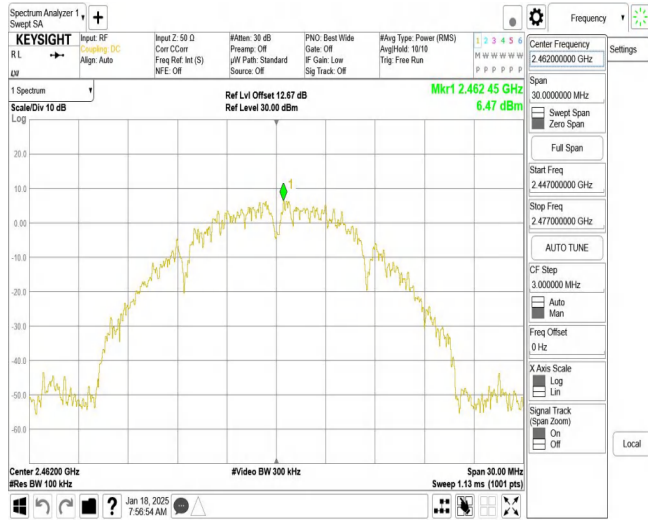
11B_Ant1_2462_0~Reference
