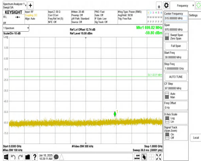
11AX20MIMO_Ant2_2412_30~1000
