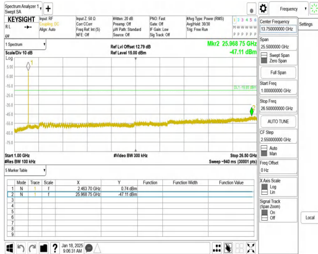
11N20MIMO_Ant2_2462_1000~26500
