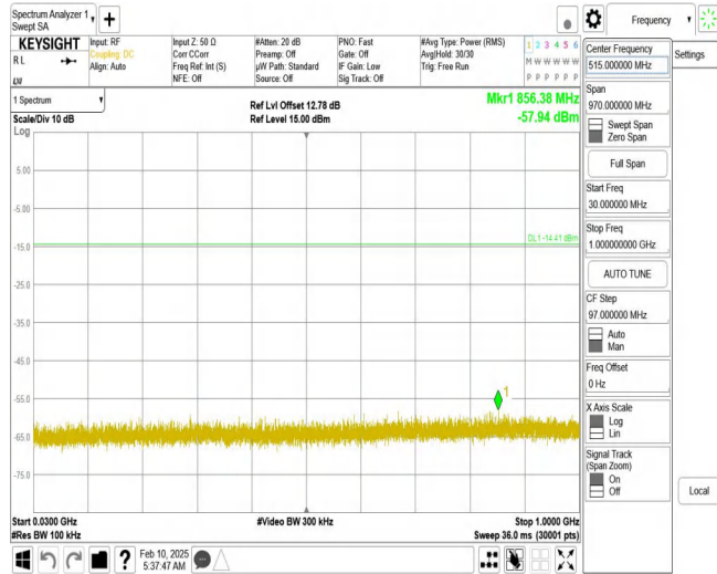
11B_Ant2_2437_30~1000
