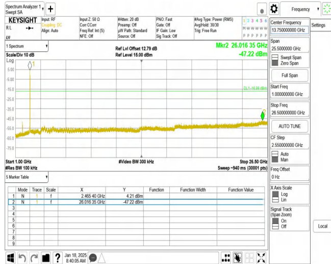
11G_Ant2_2462_1000~26500
