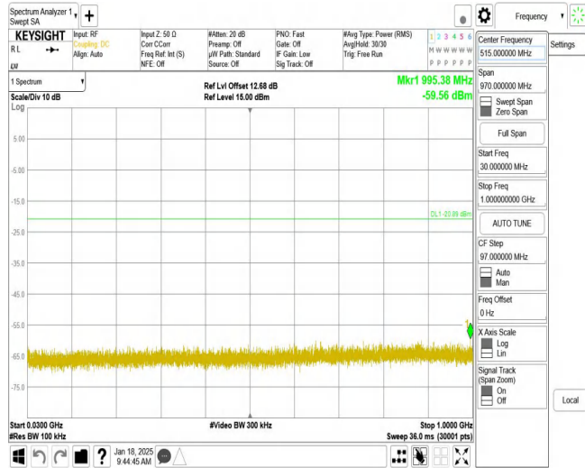
11N40MIMO_Ant1_2437_30~1000
