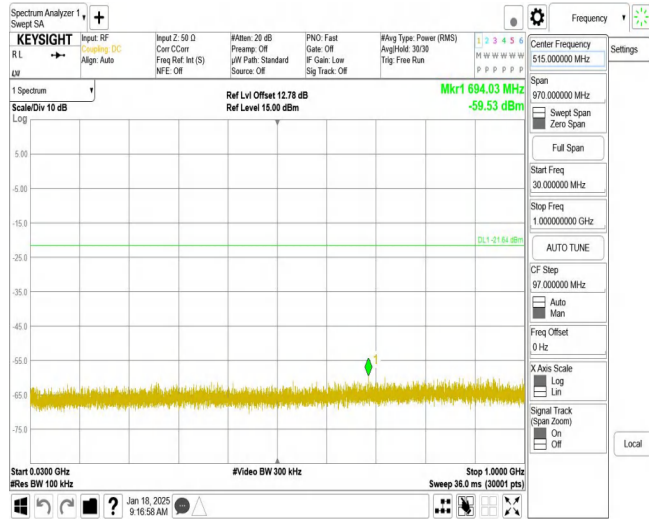
11N40MIMO_Ant2_2422_30~1000
