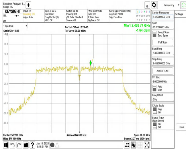
11N40MIMO_Ant2_2422_0~Reference
