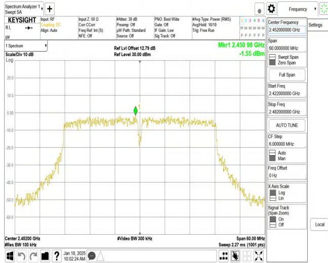
11N40MIMO_Ant2_2452_0~Reference
