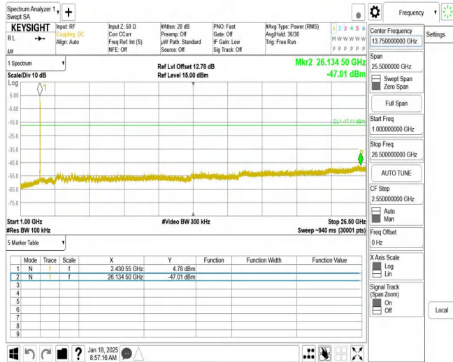
11N20MIMO_Ant2_2437_1000~26500
