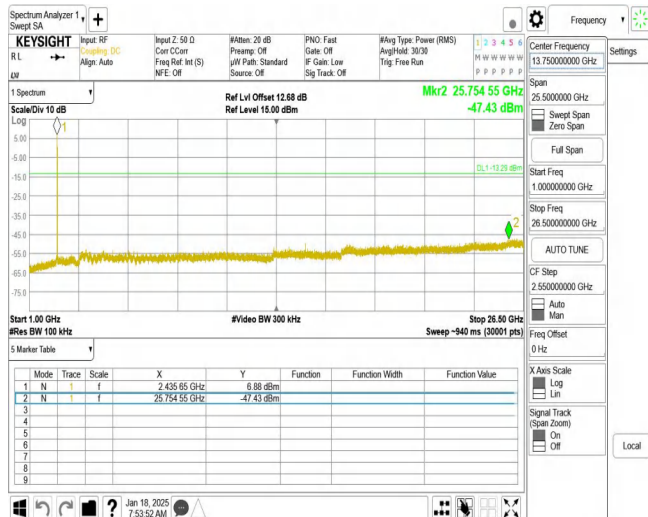
11B_Ant1_2437_1000~26500
