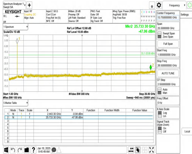
11N40MIMO_Ant1_2437_1000~26500
