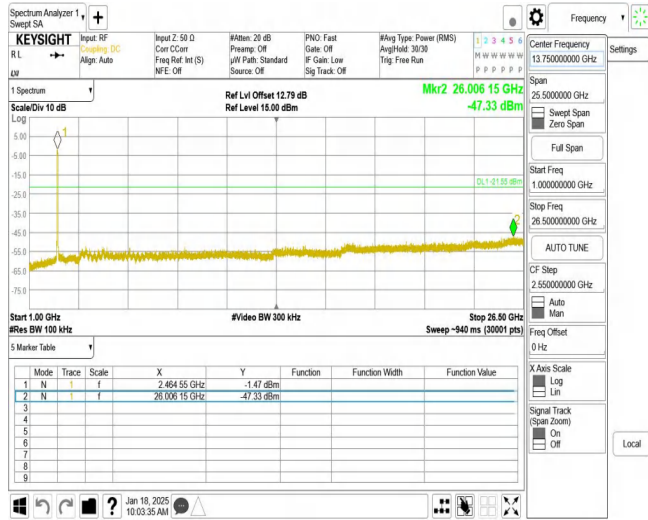
11N40MIMO_Ant2_2452_1000~26500
