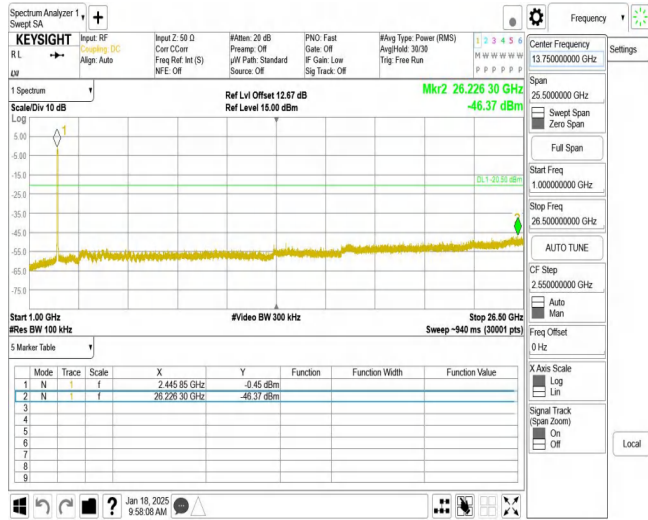
11N40MIMO_Ant1_2452_1000~26500
