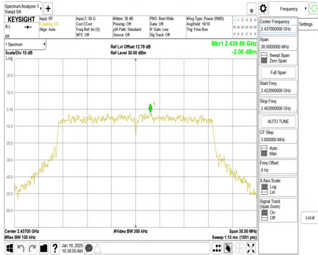
11AX20MIMO_Ant2_2437_0~Reference
