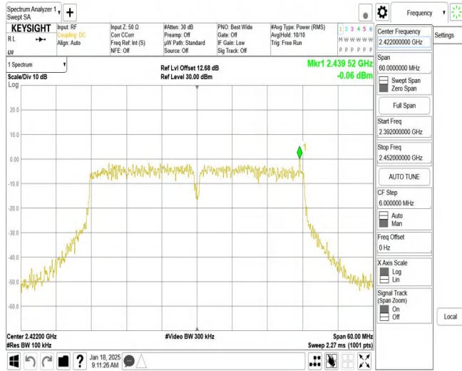
11N40MIMO_Ant1_2422_0~Reference
