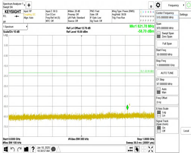
11AX20MIMO_Ant2_2437_30~1000
