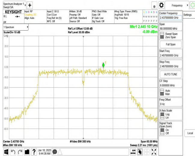
11N40MIMO_Ant1_2437_0~Reference
