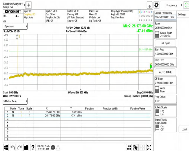
11B_Ant2_2462_1000~26500
