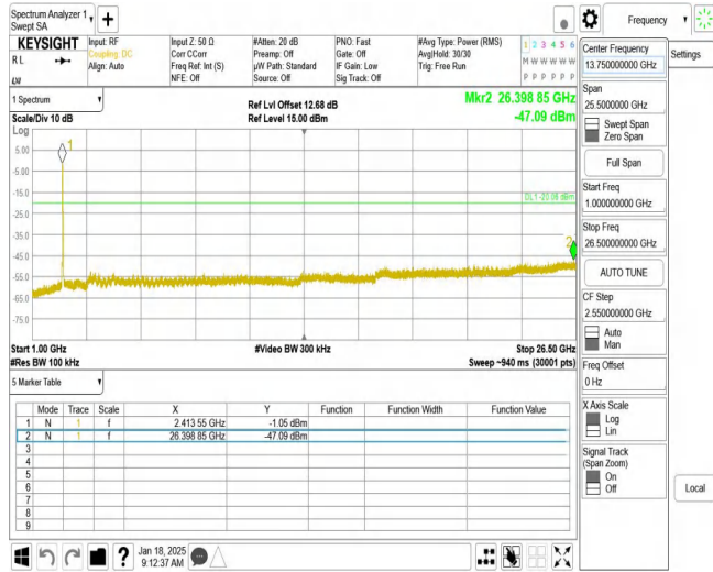
11N40MIMO_Ant1_2422_1000~26500
