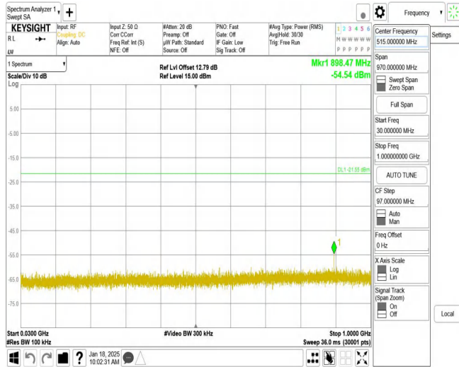
11N40MIMO_Ant2_2452_30~1000
