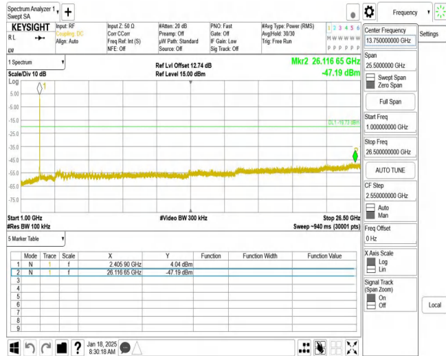
11G_Ant2_2412_1000~26500
