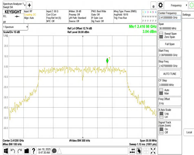
11N20MIMO_Ant2_2412_0~Reference
