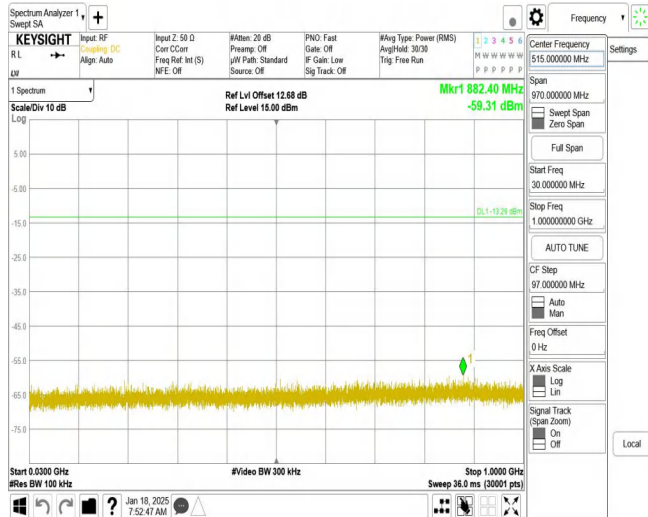
11B_Ant1_2437_30~1000
