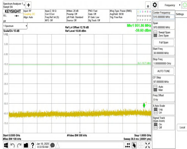
11G_Ant2_2437_30~1000
