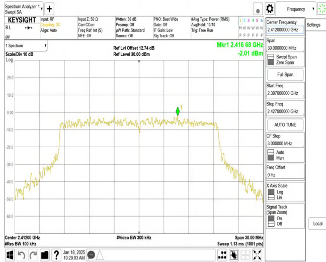
11AX20MIMO_Ant2_2412_0~Reference
