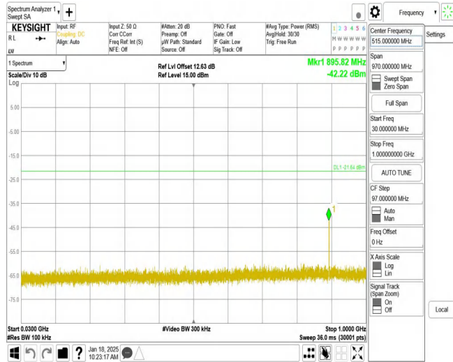
11AX20MIMO_Ant1_2412_30~1000
