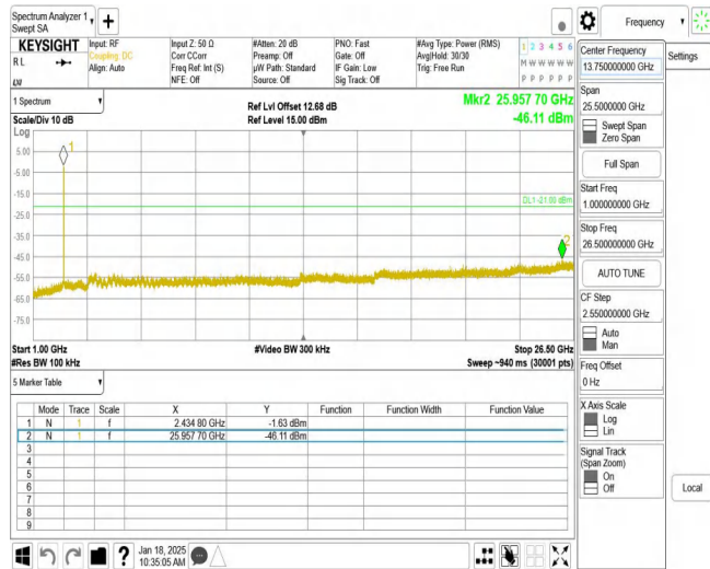
11AX20MIMO_Ant1_2437_1000~26500
