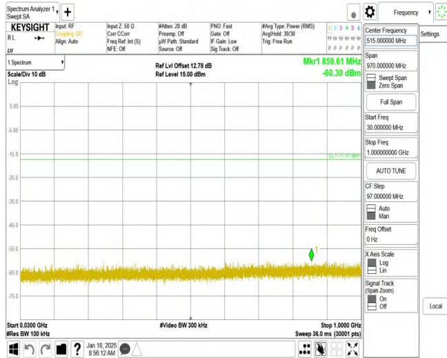
11N20MIMO_Ant2_2437_30~1000
