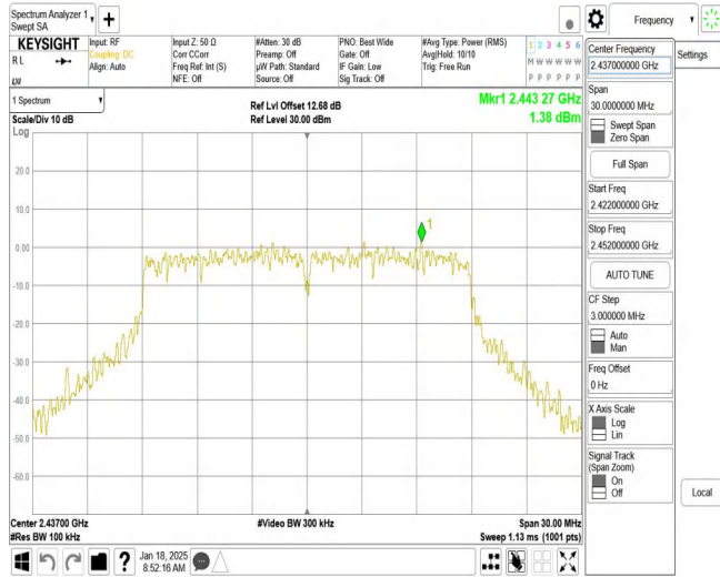
11N20MIMO_Ant1_2437_0~Reference
