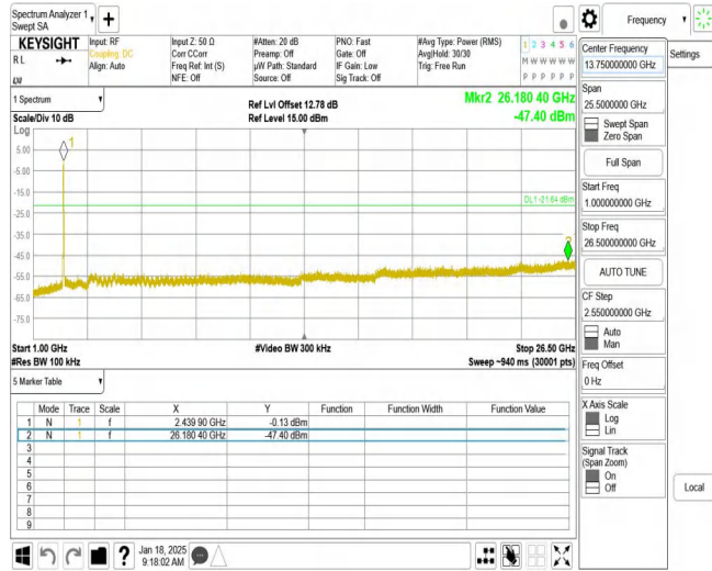
11N40MIMO_Ant2_2422_1000~26500
