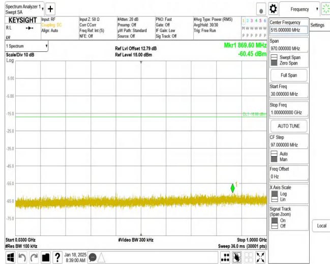
11G_Ant2_2462_30~1000
