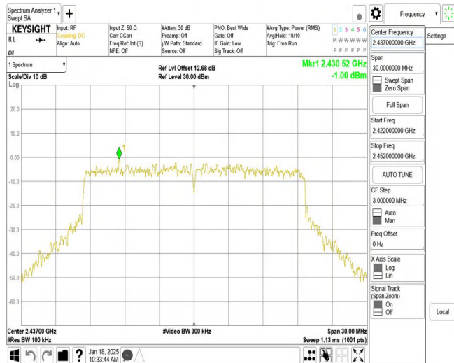
11AX20MIMO_Ant1_2437_0~Reference
