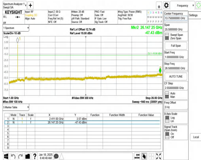
11N20MIMO_Ant2_2412_1000~26500
