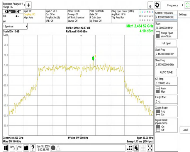
11N20MIMO_Ant1_2462_0~Reference
