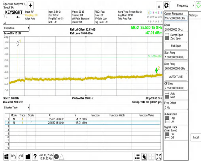
11AX20MIMO_Ant1_2412_1000~26500
