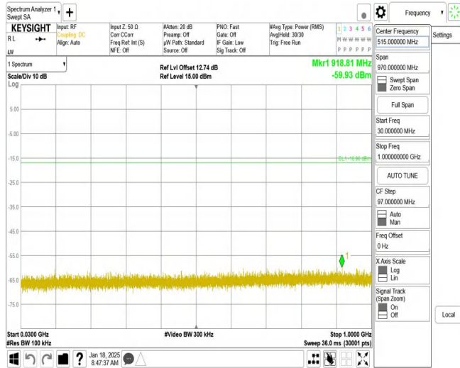
11N20MIMO_Ant2_2412_30~1000
