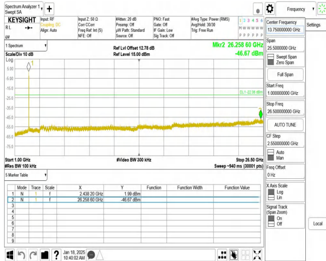
11AX20MIMO_Ant2_2437_1000~26500
