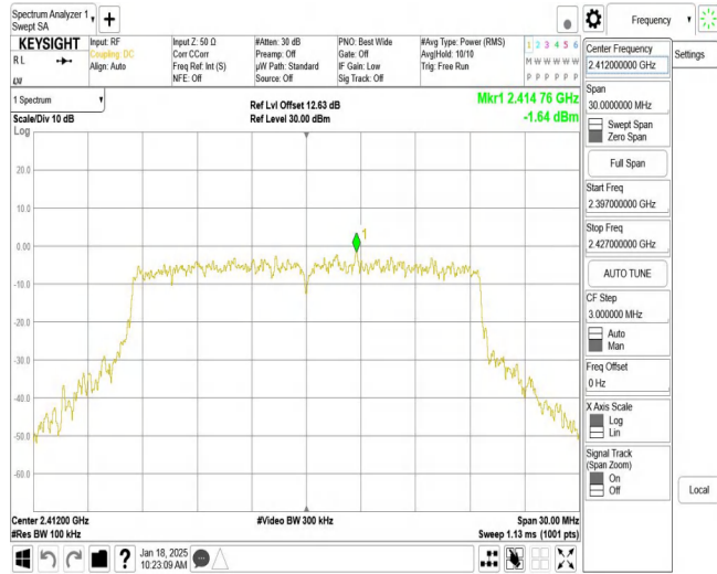
11AX20MIMO_Ant1_2412_0~Reference
