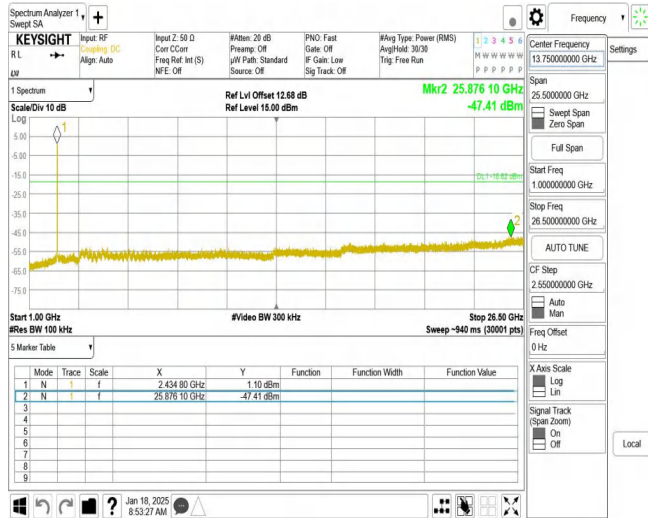
11N20MIMO_Ant1_2437_1000~26500
