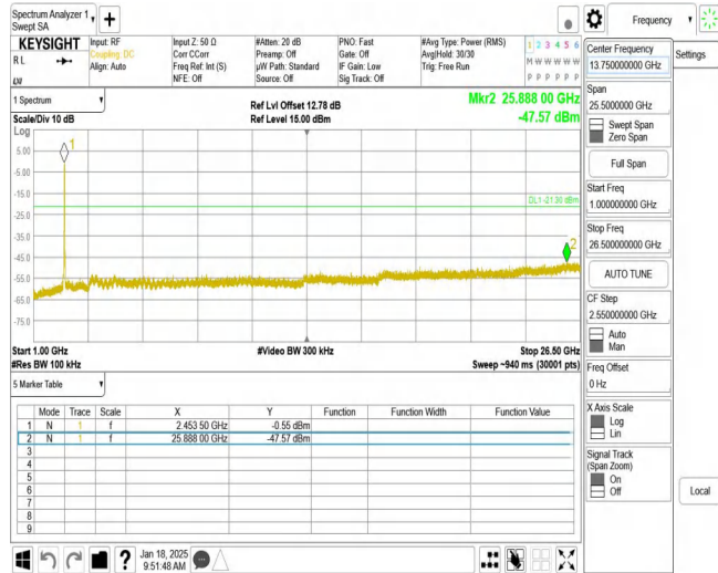
11N40MIMO_Ant2_2437_1000~26500
