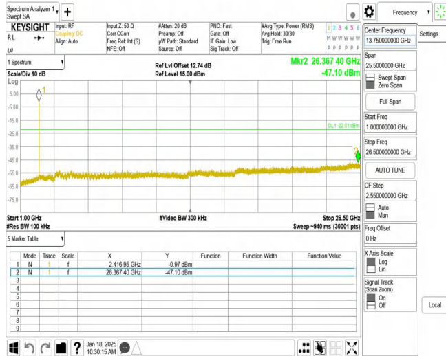
11AX20MIMO_Ant2_2412_1000~26500
