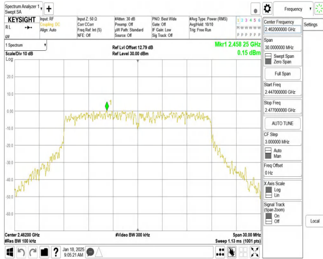
11N20MIMO_Ant2_2462_0~Reference
