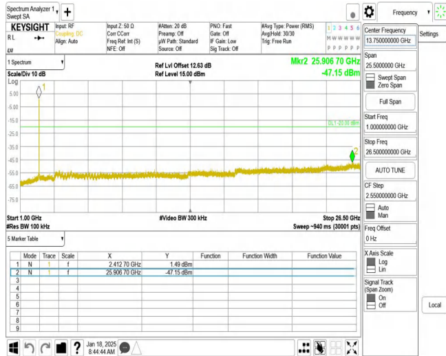
11N20MIMO_Ant1_2412_1000~26500
