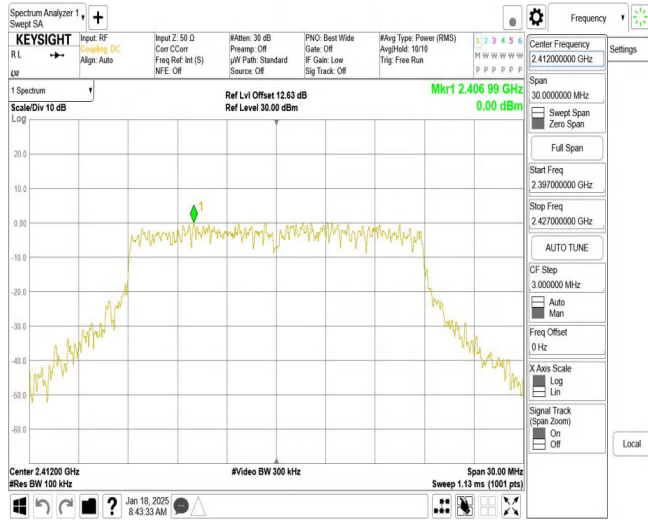
11N20MIMO_Ant1_2412_0~Reference
