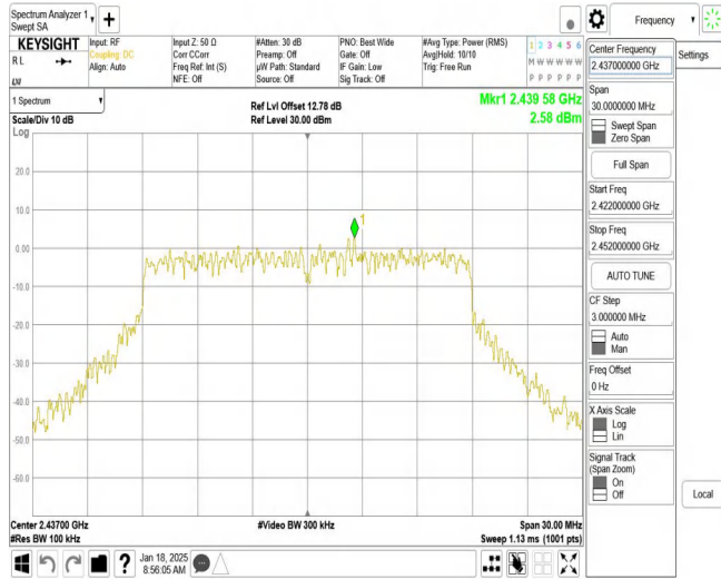
11N20MIMO_Ant2_2437_0~Reference
