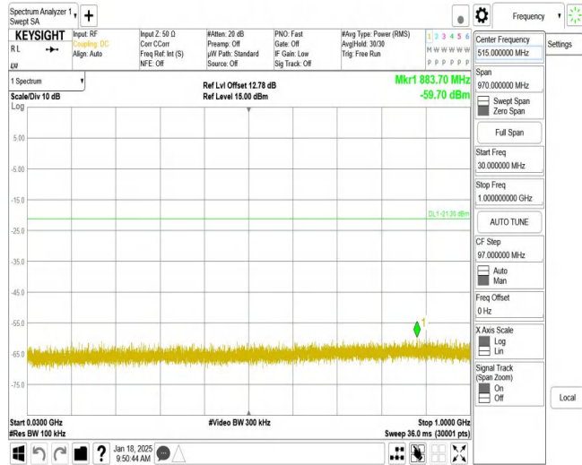
11N40MIMO_Ant2_2437_30~1000
