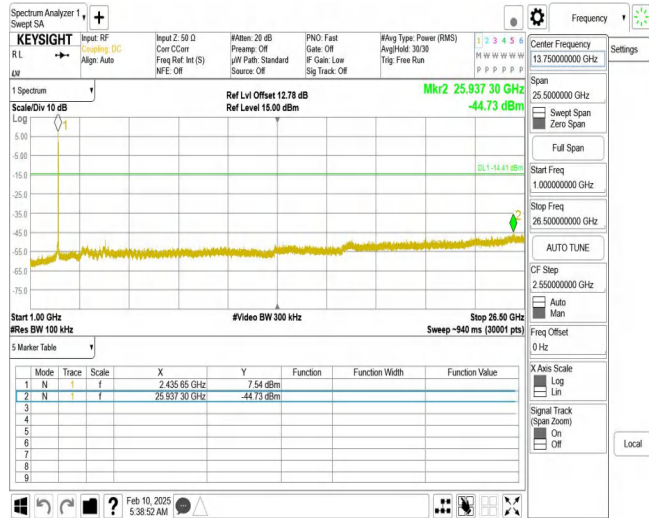
11B_Ant2_2437_1000~26500
