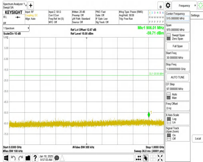
11N40MIMO_Ant1_2452_30~1000
